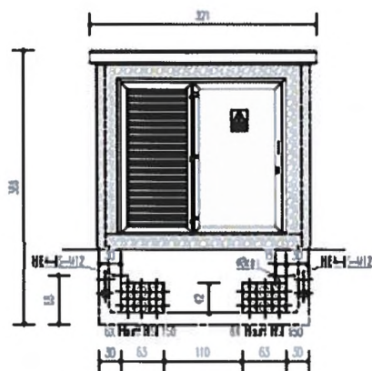
Aanzicht B
