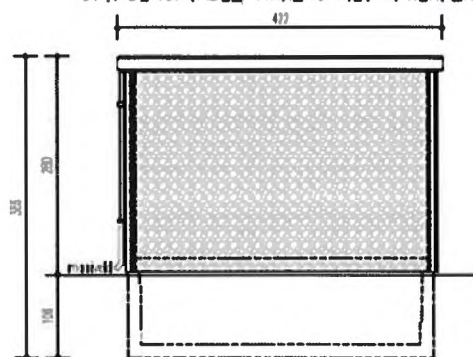
Aanzicht A
