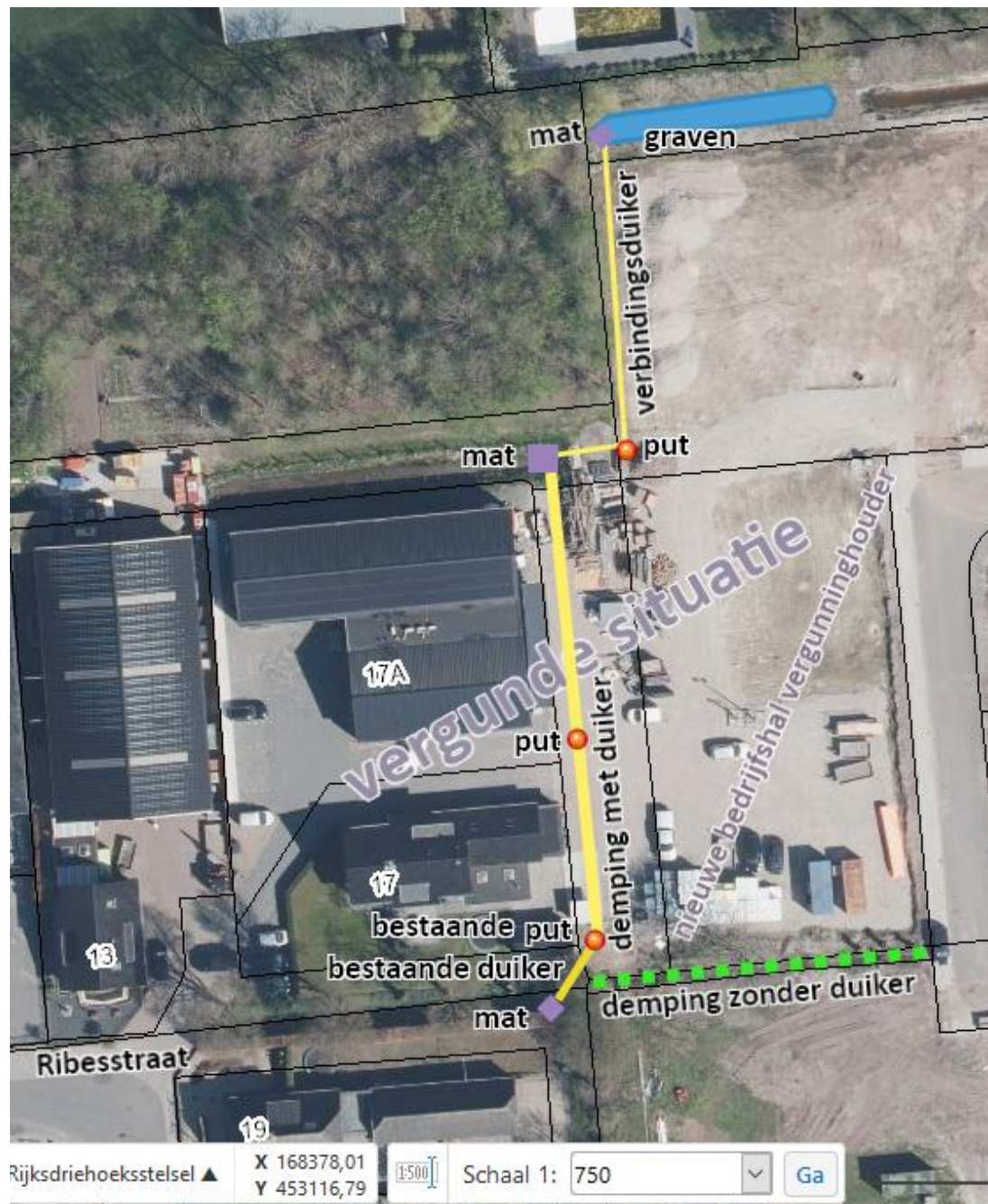
Situatietekening na voltooiing van de werkzaamheden
