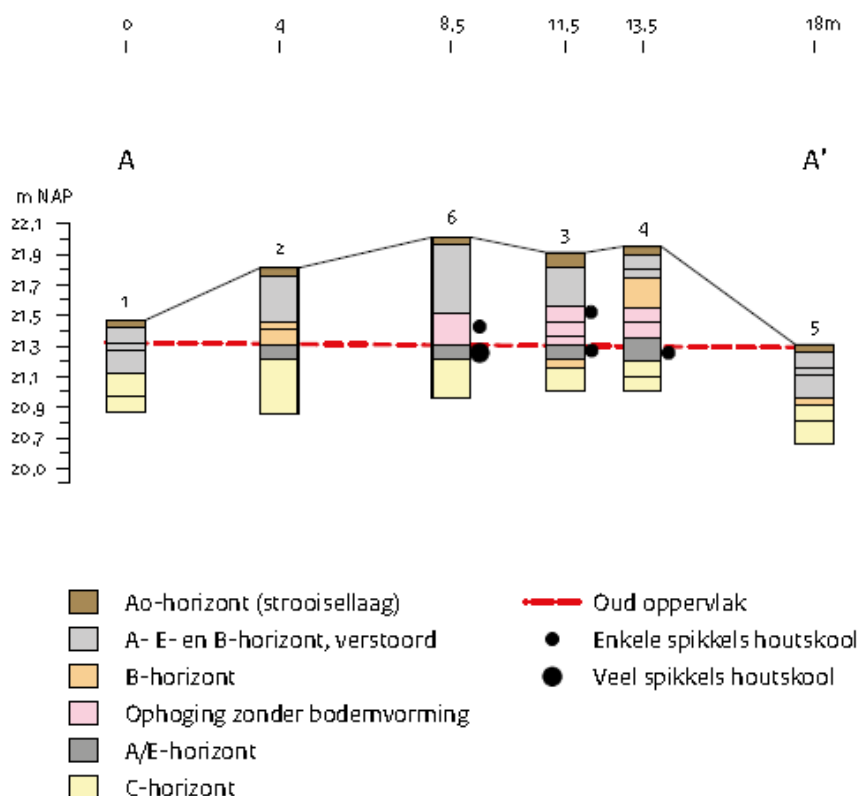
Fig. 22 Schematisch boorprofiel over de Molshoop. Het onderzoek leverde opmerkelijk veel houtskoolfragmenten van het oud oppervlak op (uit Theunissen en de Kort 2017).
