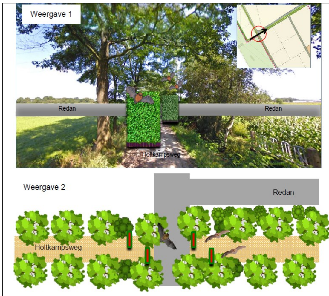
Figuur 5. Een schematische weergave van de zogenaamde hop-over die geplaatst wordt tussen deelgebied noord en centraal, bij de doorsnijding van de Holtkampsweg te Groenlo. De schermen zijn minimaal 2 meter hoog (twee van één meter op elkaar) en 4 meter lang en aan beide zijden begroeid met klimop en omgeven door struiken. Aan beide zijden van de doorsnijding worden twee schermen om en om geplaatst (4 locaties totaal). Op die manier wordt beoogd het lijnelement intact te houden en vleermuizen die gebruik maken van de laan als vliegroute te 'stuwen' voor een veilige oversteek. Ook kunnen voetgangers en fietsers op deze manier gewoon gebruik maken van de Holtkampsweg. De afstand tussen de kronen van de bomen boven de nieuwe ontsluitingsweg is maximaal 5 meter.
