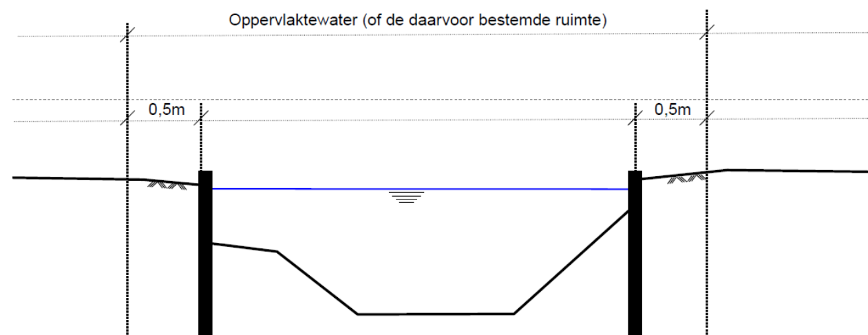
Figuur 1.4. Afbakening waterbeheergebied bij beschoeiide oevers die niet zijn vastgelegd in de legger.
