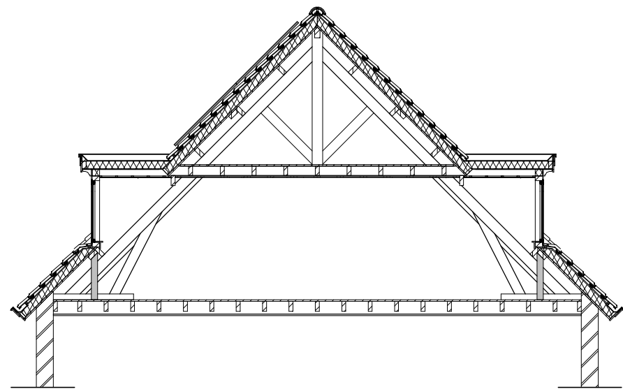
doorsnede kap BSO 1:100
