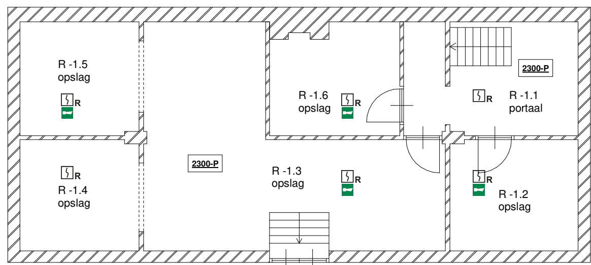
kelder 1:100
