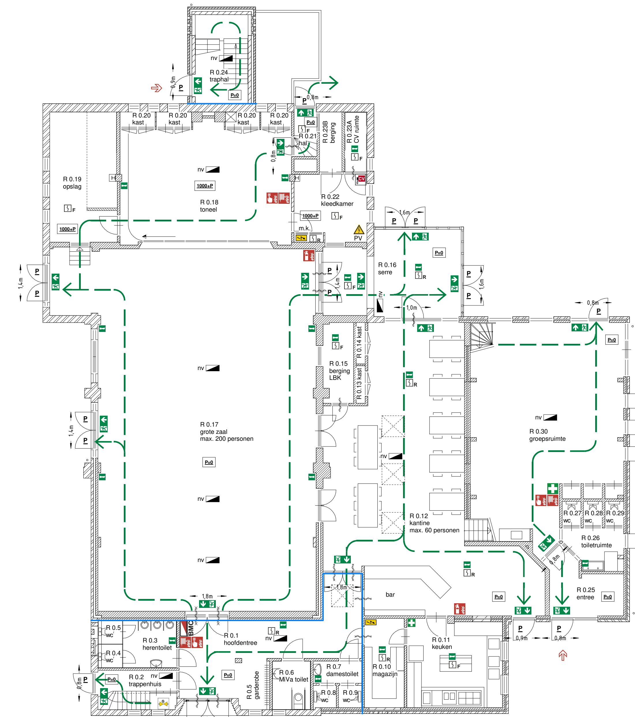
begane grond 1:100
