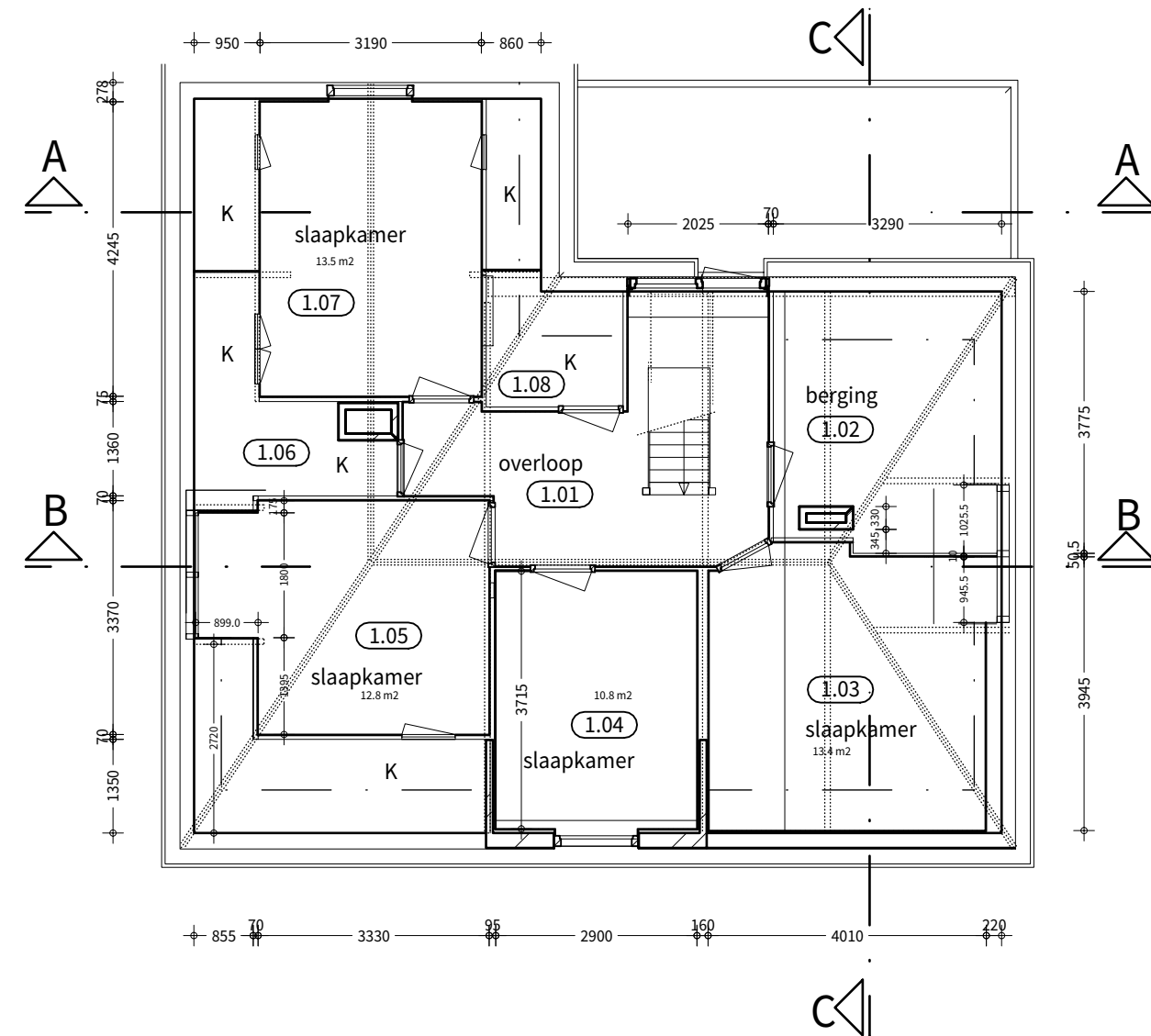
VERDIEPING bestaand P = 3500+
