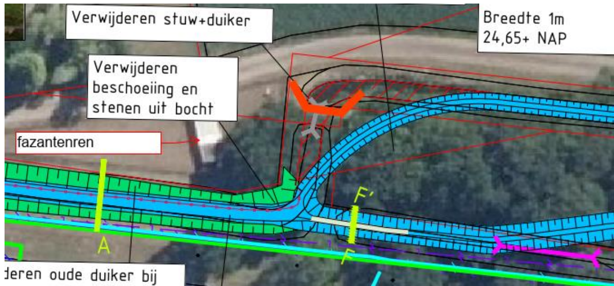
Figuur 19: Verwijderen stuw 253P, duiker en klinkers in bocht
