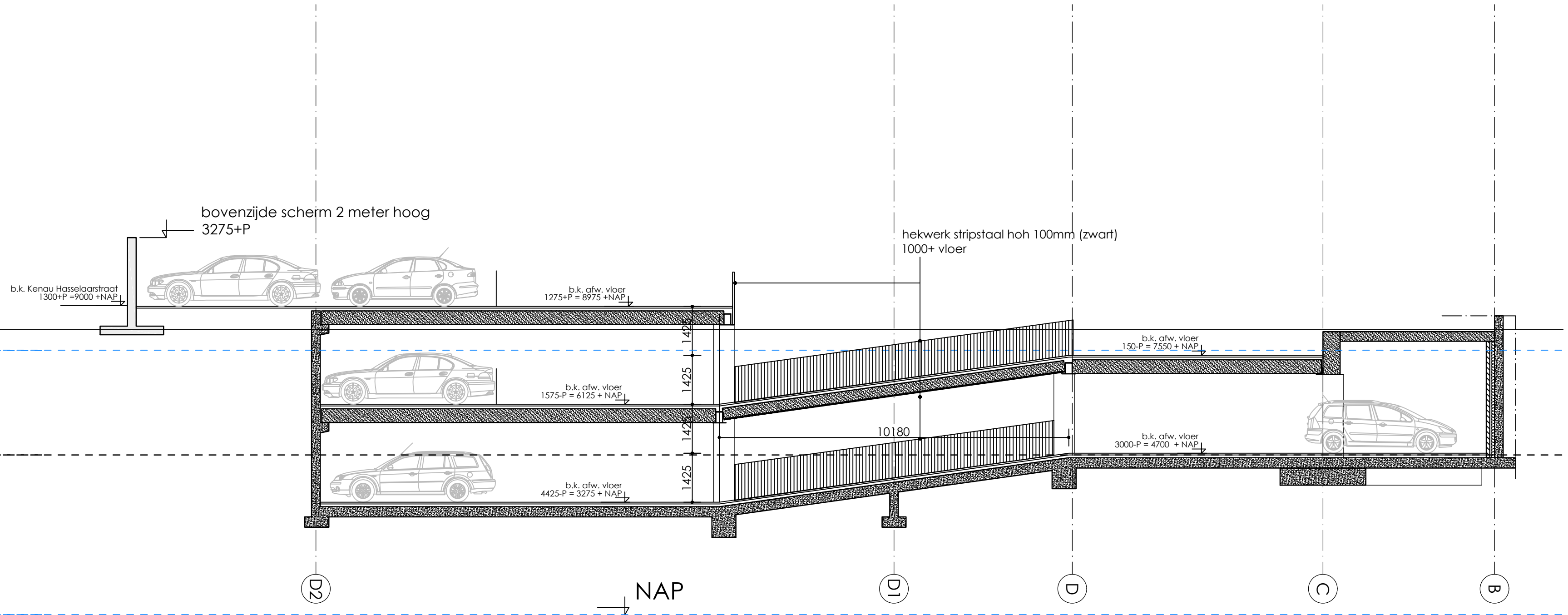
Doorsnede DD 1:100
