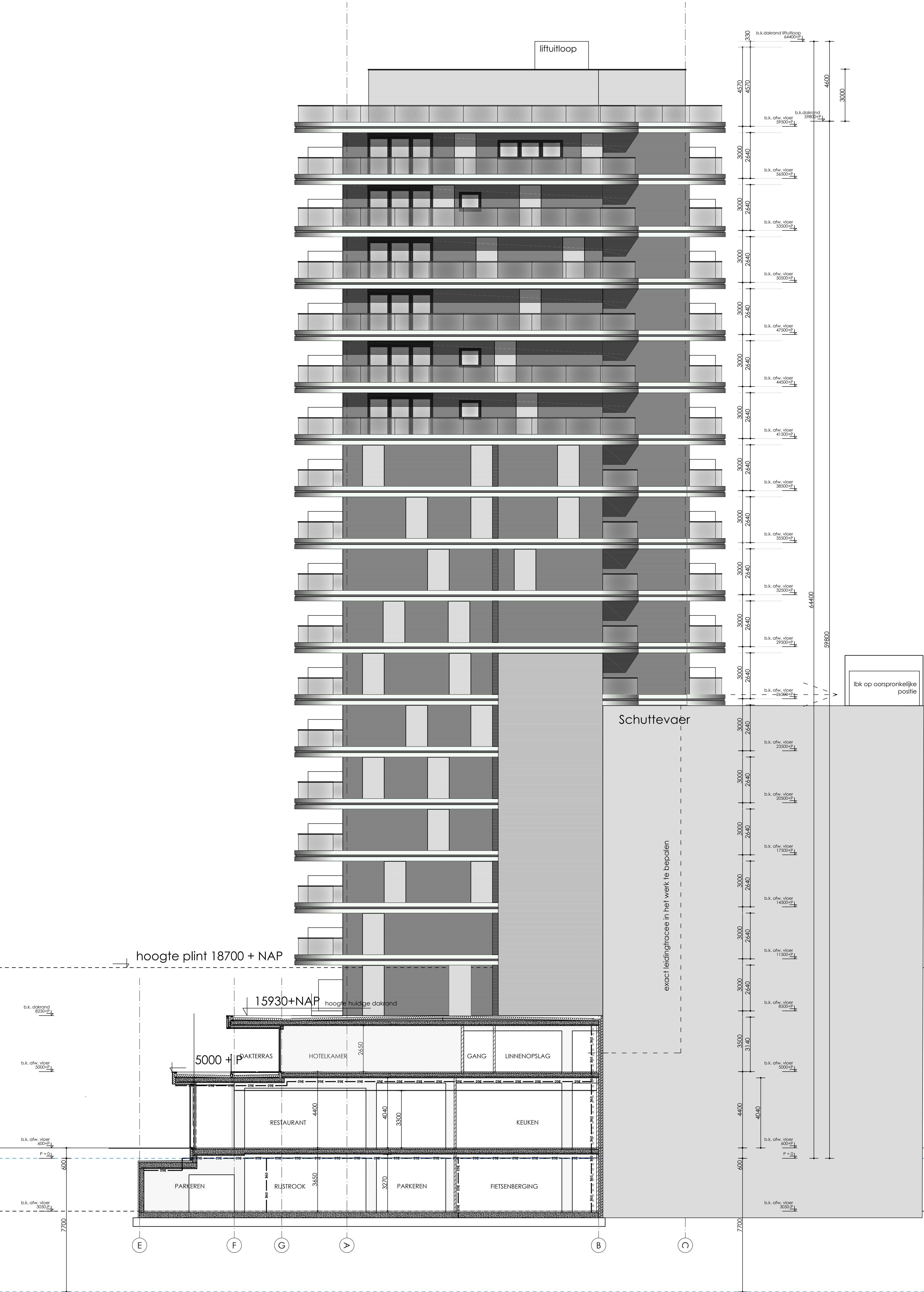
Doorsnede CC 1:100
