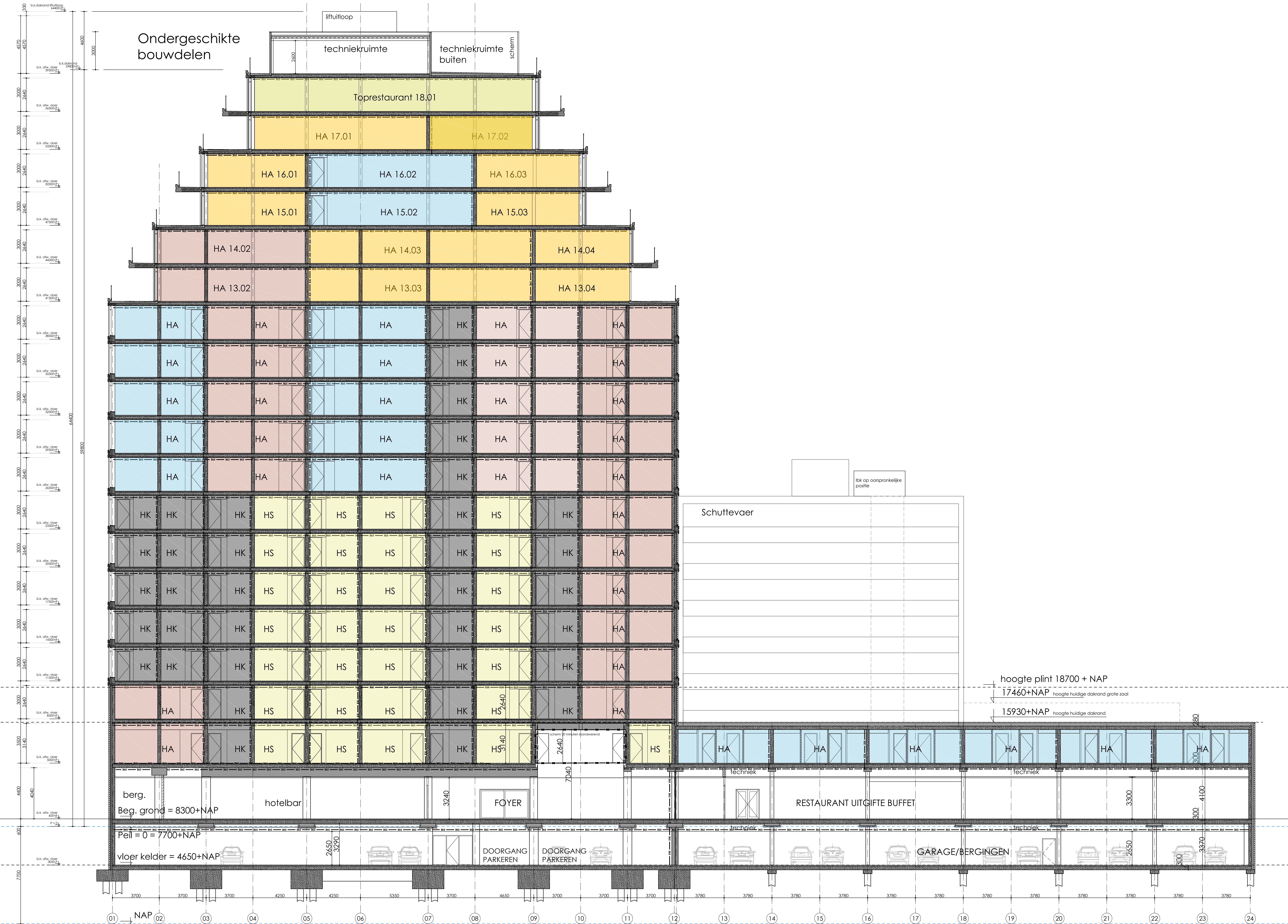
Doorsnede BB 1:100
