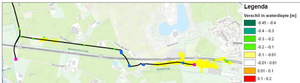
Figuur 5-4 Vershilkaart inundatiediepte huidige en beoogde situatie (deze afbeelding geeft het verschil in inundatiediepte tussen de huidige en de beoogde situatie in landelijk gebied weer; bv. de gele vlakken geven een afname van de waterdiepte met 0,01 tot 0,1 m weer)
