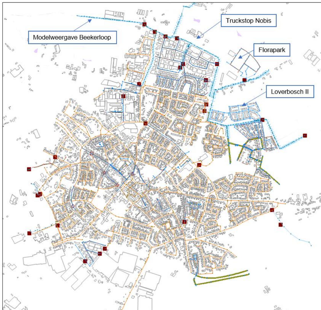
Figuur 2 - Impressie van het rioleringsmodel en de vier aanpassingen die hebben plaatsgevonden. De watergangen van de Beekerloop zijn in het lichtblauw weergegeven. De oranje, blauwe en bruine lijnen representeren respectievelijk gemengde, hemelwater- en vuilwaterriolering. De zwarte blokjes tonen de overstorten en stuwen. De kern Ommel is niet zichtbaar in dit overzicht.
