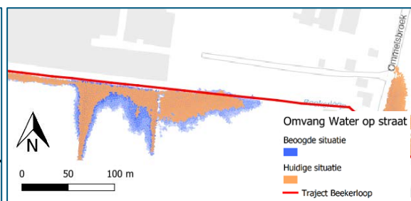
Figuur 10 – Verschil in omvang na traject 7
