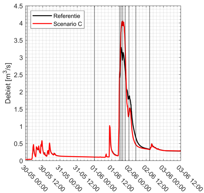
Figure 2-2: Afvoergolven voor het Scenario Referentie en C. Deze worden opgelegd op de bovenstroomse rand op de Beekerloop. Met stippellijnen zijn de tijdstippen aangegeven waarop langsdoorsnedes zijn gemaakt.
