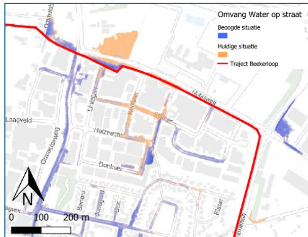
Figuur 8 – Verschil in omvang water op straat nabij Nobisweg
