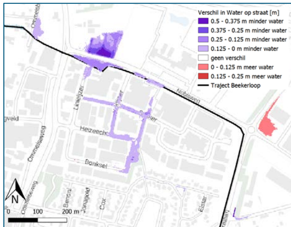
Figuur 7 – Verschil in waterdiepte nabij Nobisweg
