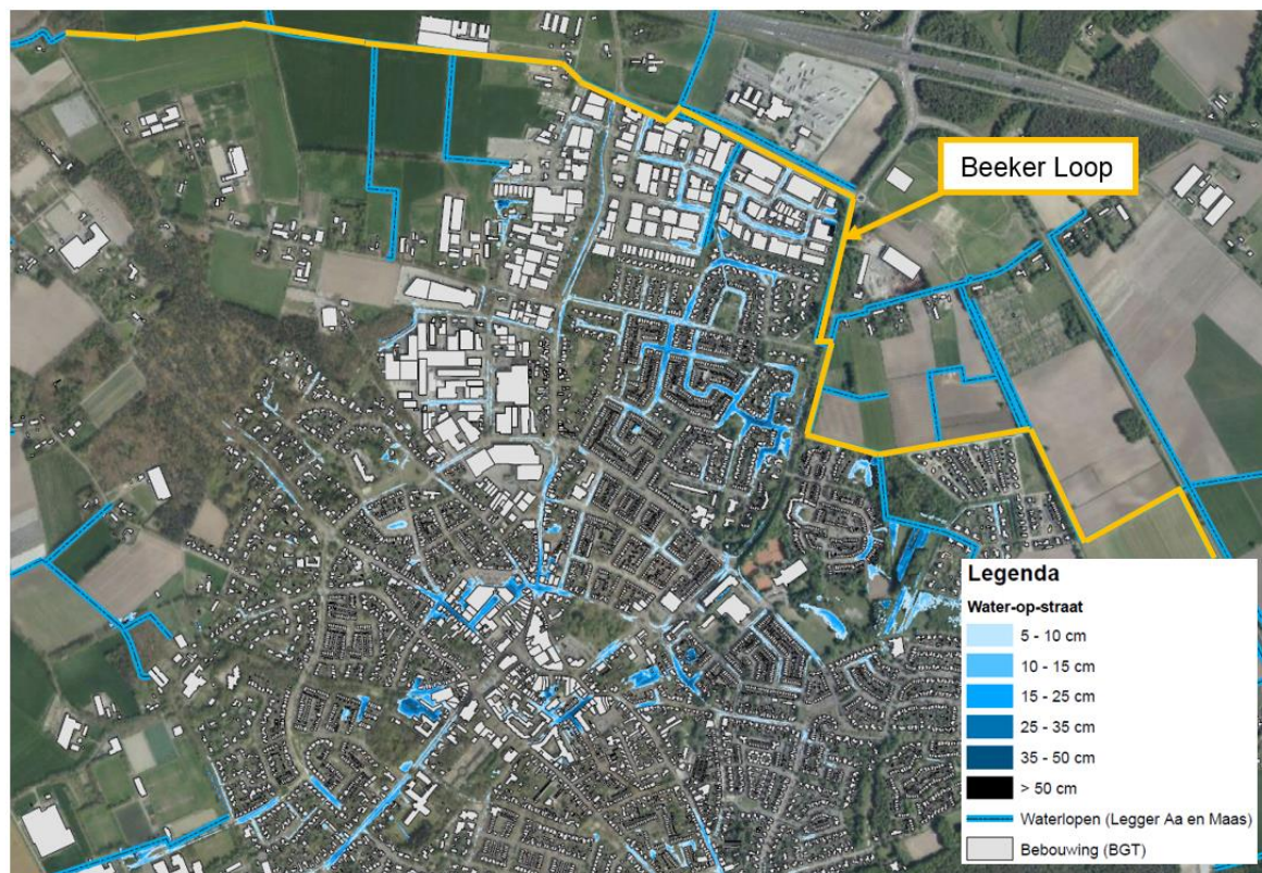
Figuur 1 – Water-op-sstraat kaart die is opgesteld om de wateroverlast in 2016 te benaderen. In het geel is de Beekerloop gearceerd, waar door uitwisseling tussen riolering en oppervlaktewater hoge waterstanden hebben plaatsgevonden. De Beekerloop stroomt in het figuur van rechts naar links.
