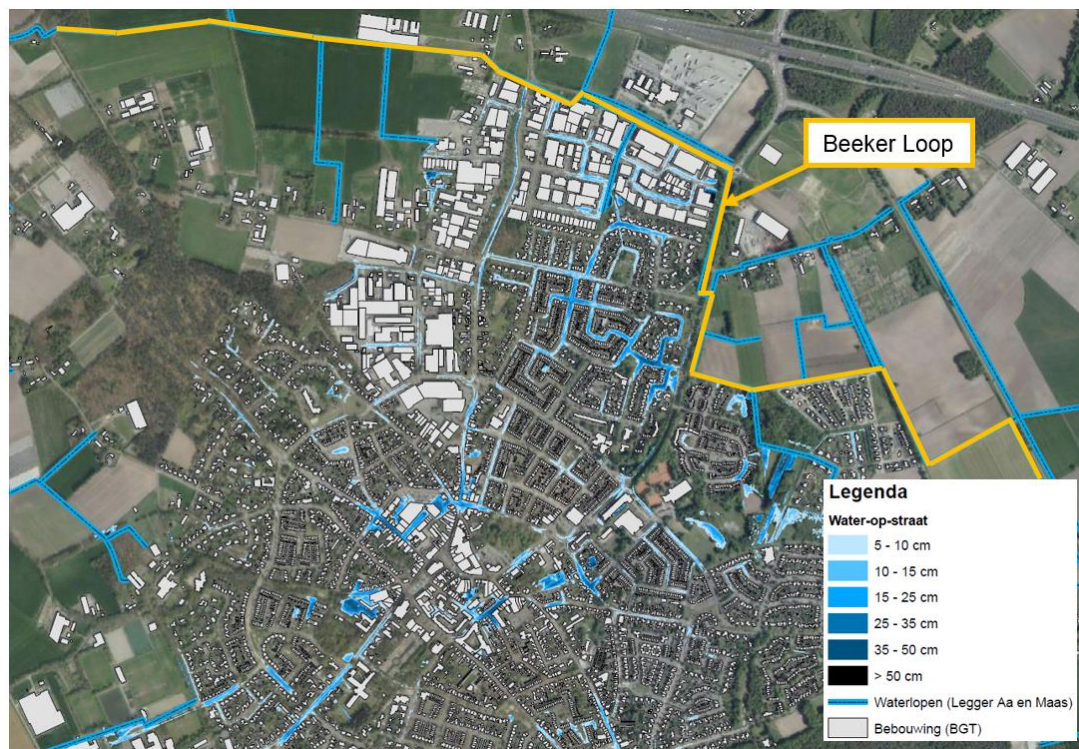
Figuur 2-2 Water-op-sstraat kaart die is opgesteld om de wateroverlast in 2016 te benaderen. In het geel is de Beekerloop gearceerd, waar door uitwisseling tussen riolering en oppervlaktewater hoge waterstanden hebben plaatsgevonden. De Beekerloop stroomt in het figuur van rechts naar links.
