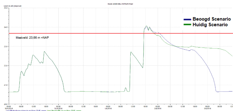
Figuur 14 - Waterdiepte Plutostraat
