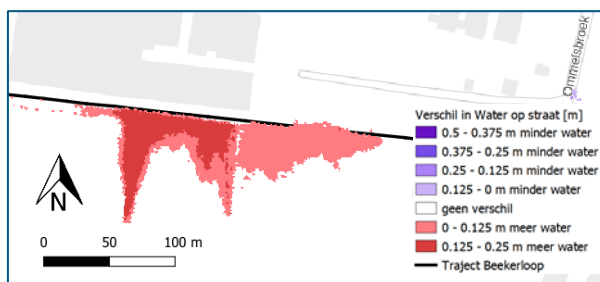
Figuur 9 – Verschil in waterdiepte na traject 7
