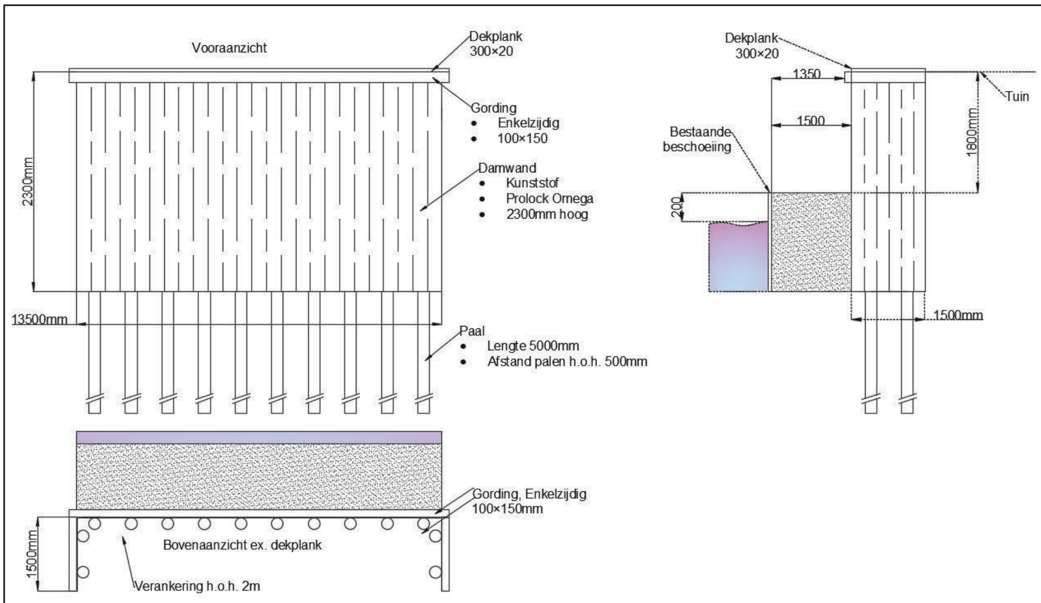
372908-C Detail en dwarsprofiel
