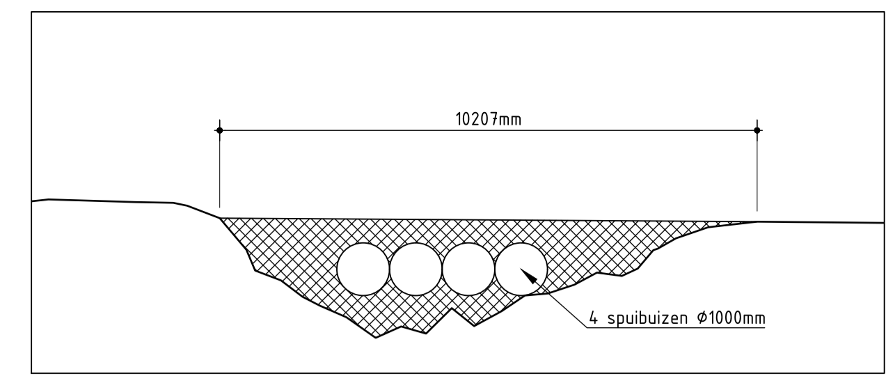
Detail 1: Schaal 1:100 Gronddammen zijn voorzien van 4x DN1000 spuikokers t.b.v. behoud waterhuishouding
