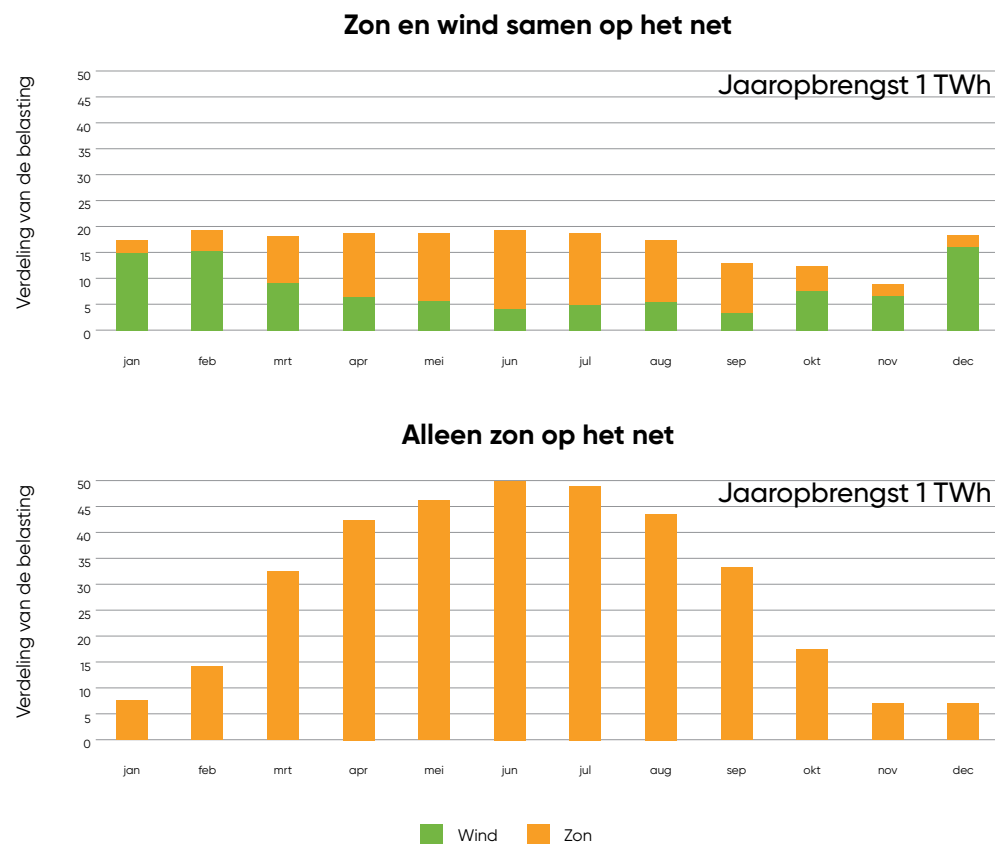
Figuur 2.6: Verhouding productie uit zon en wind. Bron: Liander, Kansenskaart E-net grootschalige opwek (2020).
