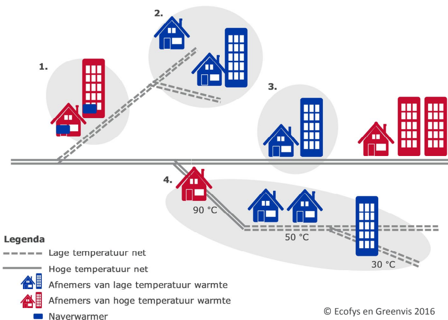
Figuur: 5.1: warmtecascade. Bron: Ecofys en Greenvis
