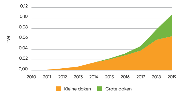
Figuur 2.11: ontwikkeling zon op grote en kleine daken. Op een groot dak passen minimaal 50 panelen (>15 kWp). Bron: De Klimaatmonitor (bewerking RES Holland Rijnland).
