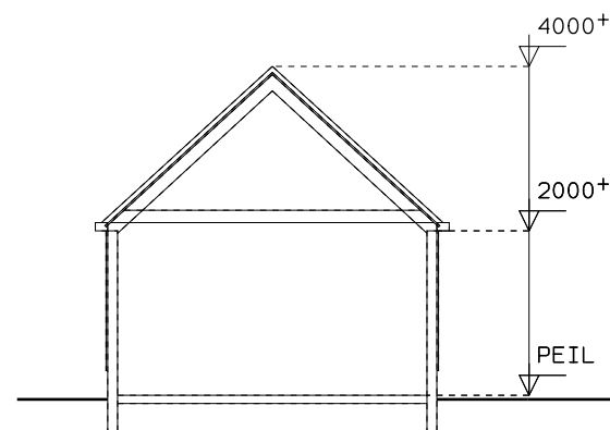
Doorsnede (bestaand)
