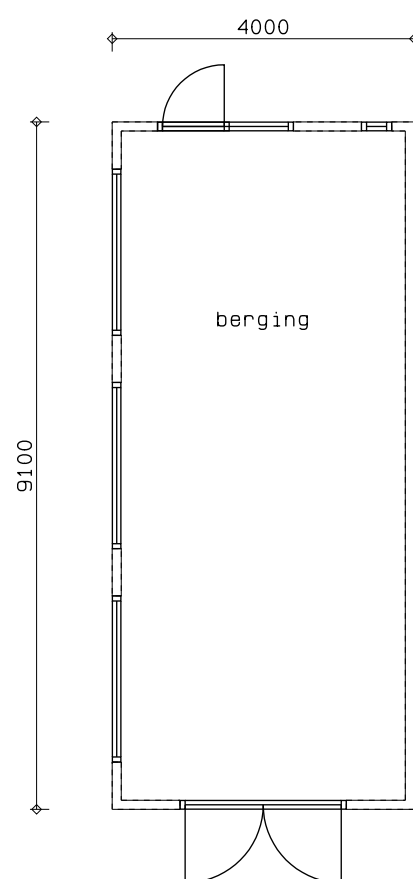
Plattegrond (bestaand)
