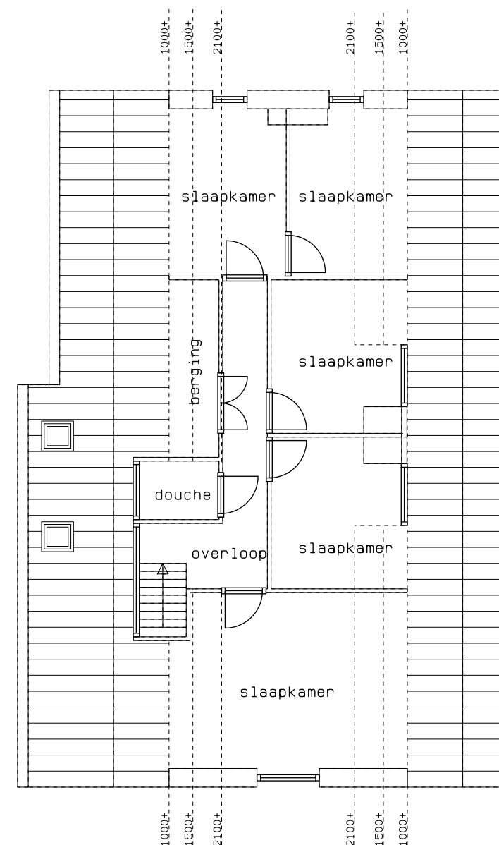
Verdieping (bestaand)
