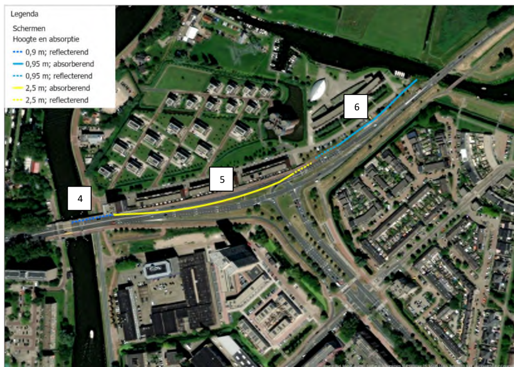
Figuur 4.3. Voorgestelde overdrachtsmaatregelen voor deelgebied 1, Oude Spoorbaan geprojecteerd op de luchtfoto van de huidige situatie.
