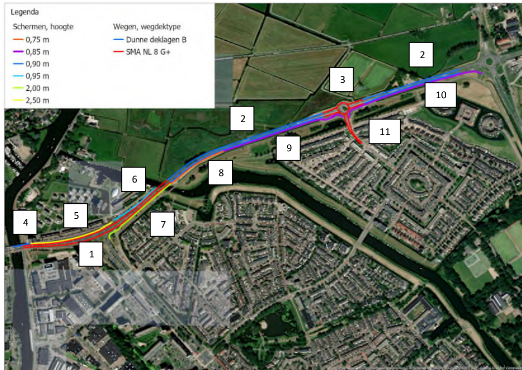
Figuur 5.1. Totaalpakket aan voorgestelde bronmaatregelen (1-3, 11) en schermmaatregelen (4-10) voor Oude Spoorbaan, Engelendaal, en Schildwacht.
