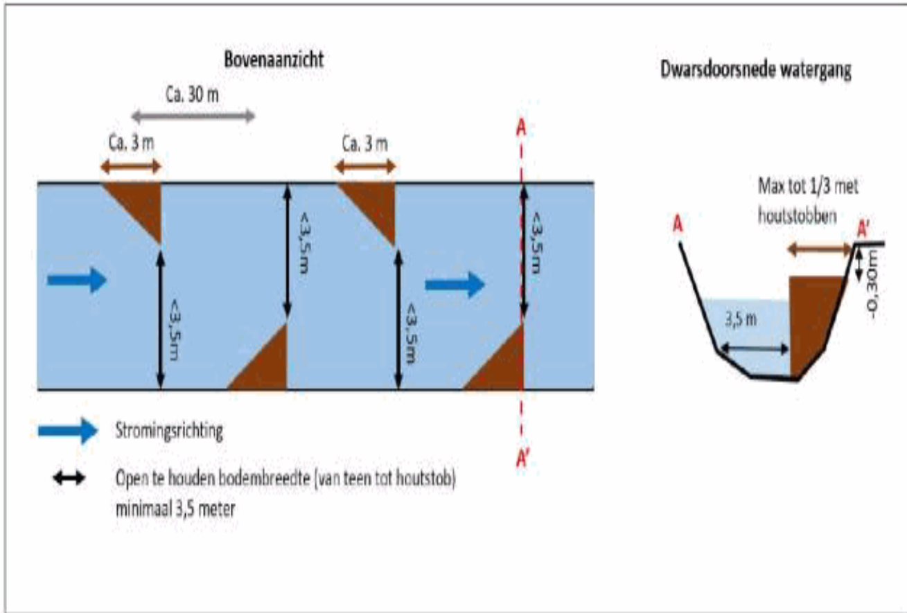
Figuur 4 Principeschets van de te plaatsen houtkribben
