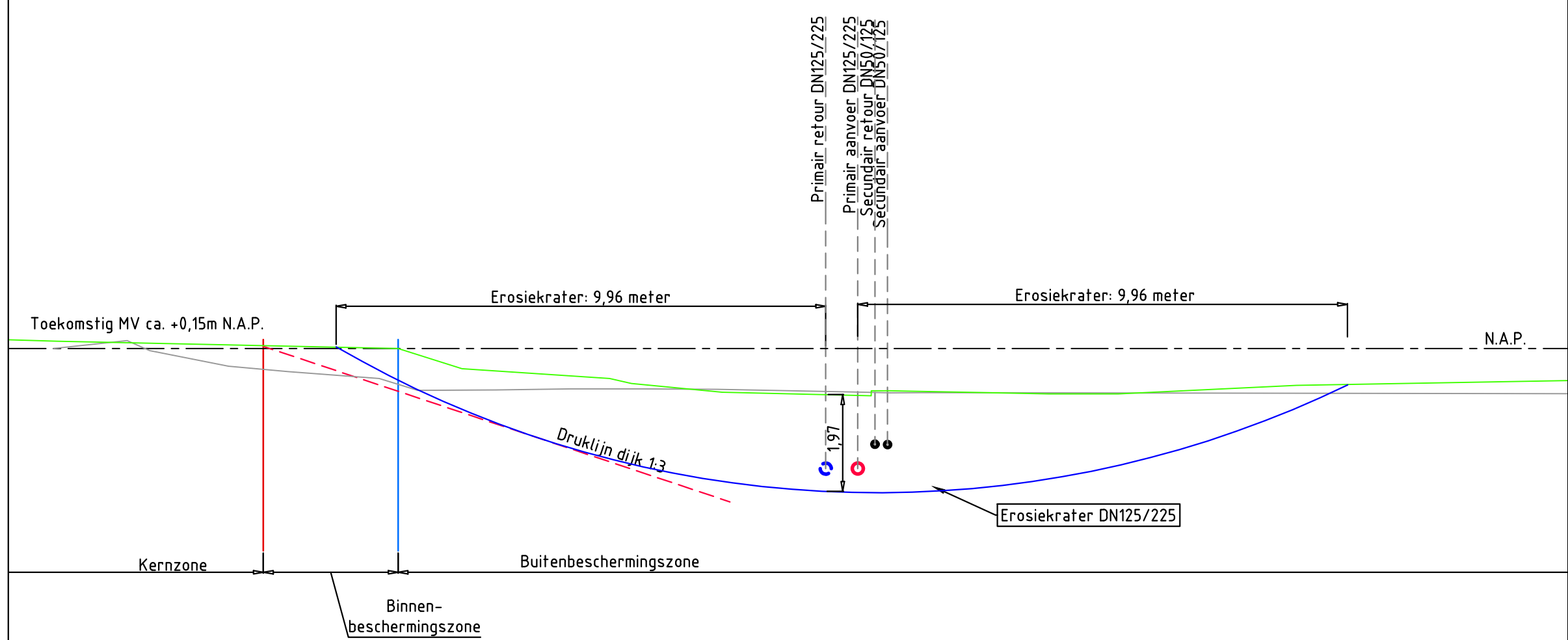
Doorsnede A-A' - Erosiekrater DN125/225
