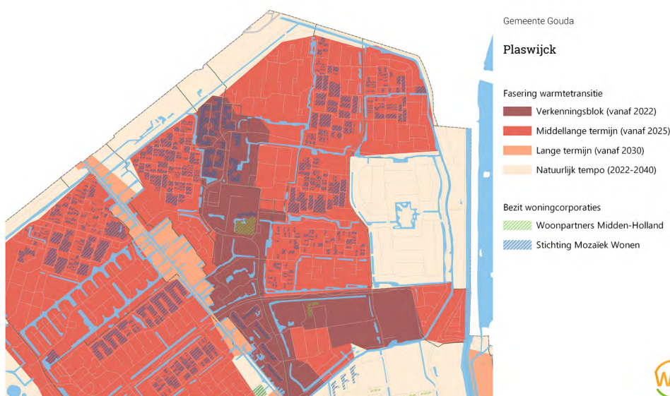
Figuur 14 Fasering warmtetransitie Plaswijck: ligging verkenningsblok
