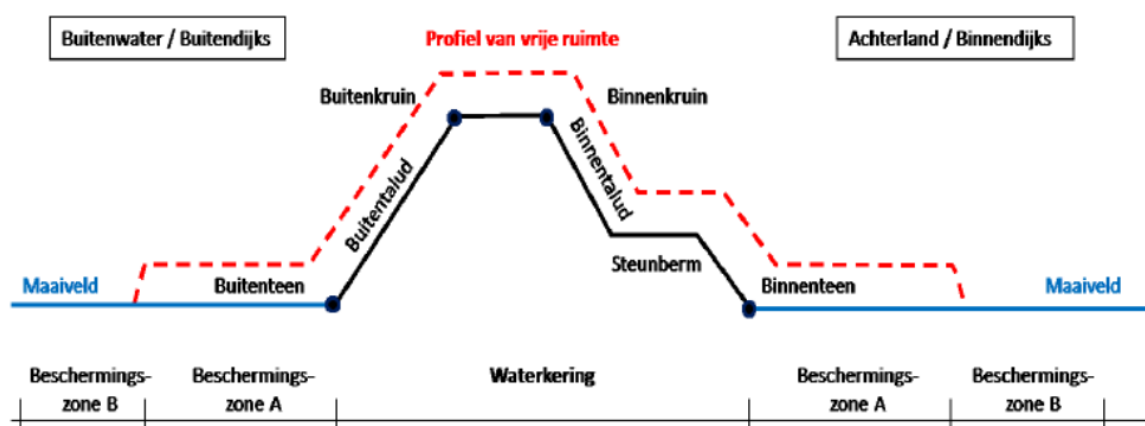
Figuur 2 Tekening principeprofiel waterkering
