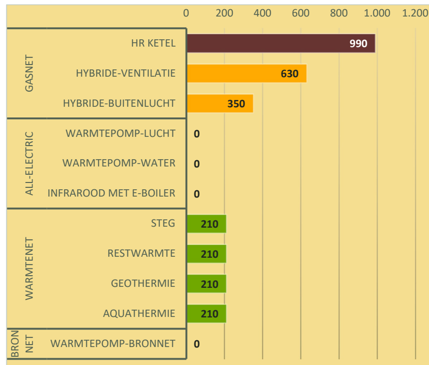
Figuur 2: Gasverbruik per techniek in m 3 /jaar, uitgesplitst naar techniek, voor een transitiegedere rijwoning 1950-1980. Gasverbruik in de elektriciteitsproductie en de hoofdbron van de STEG zijn in deze grafiek niet meegenomen.
