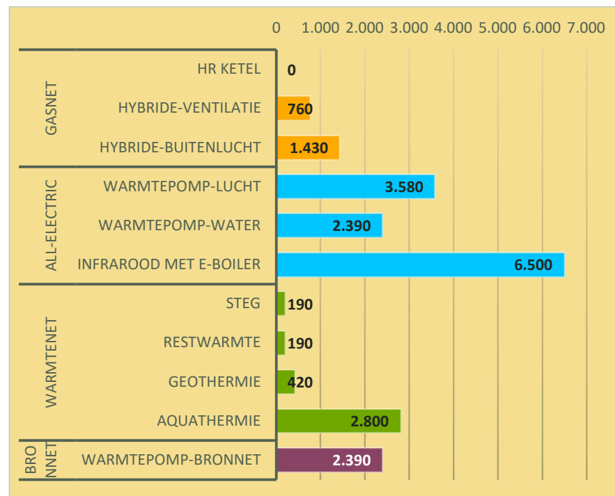
Figuur 1: Elektriciteitsverbruik per techniek in kWh/jaar, uitgesplitst naar techniek, voor een transitiegereede rijwoning 1950-1980
