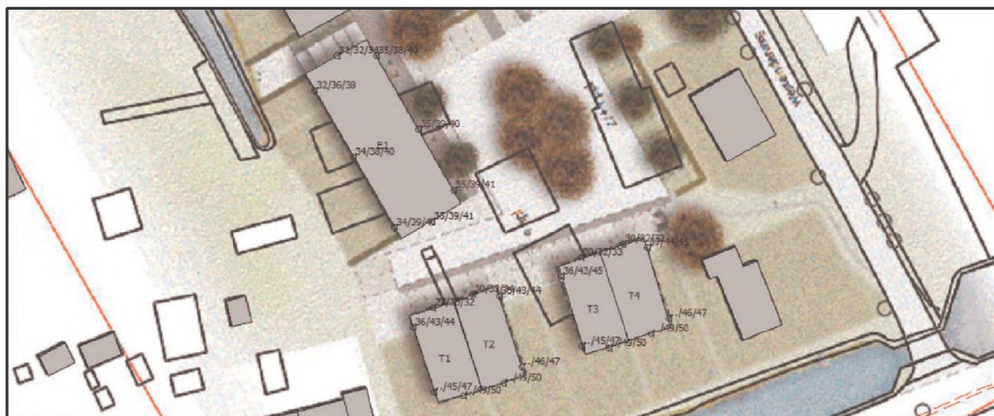
Figuur 3: Geluidsbelastingen afkomstig van de Doctor Van Noortstraat in autonome situatie (zonder rondweg)
