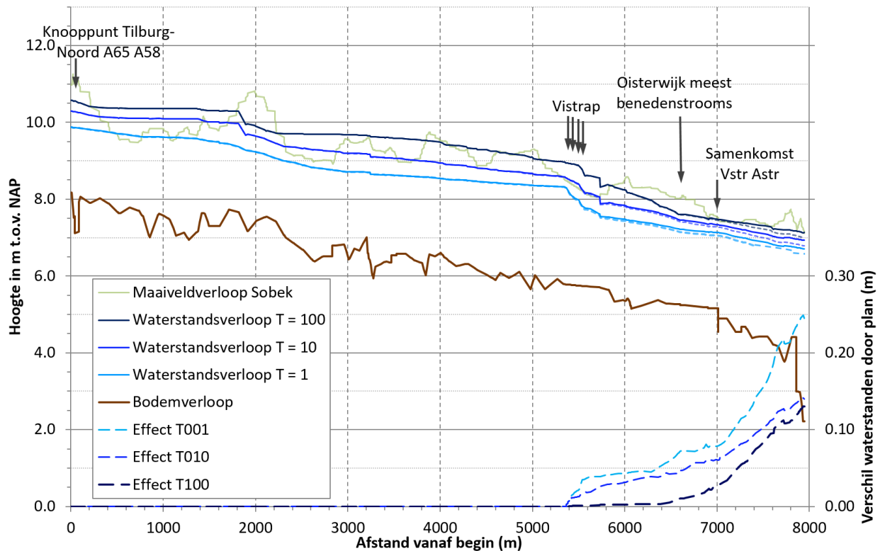
Figuur 28: Uitdemping waterstandsverhogend effect in bovenstroomse richting
