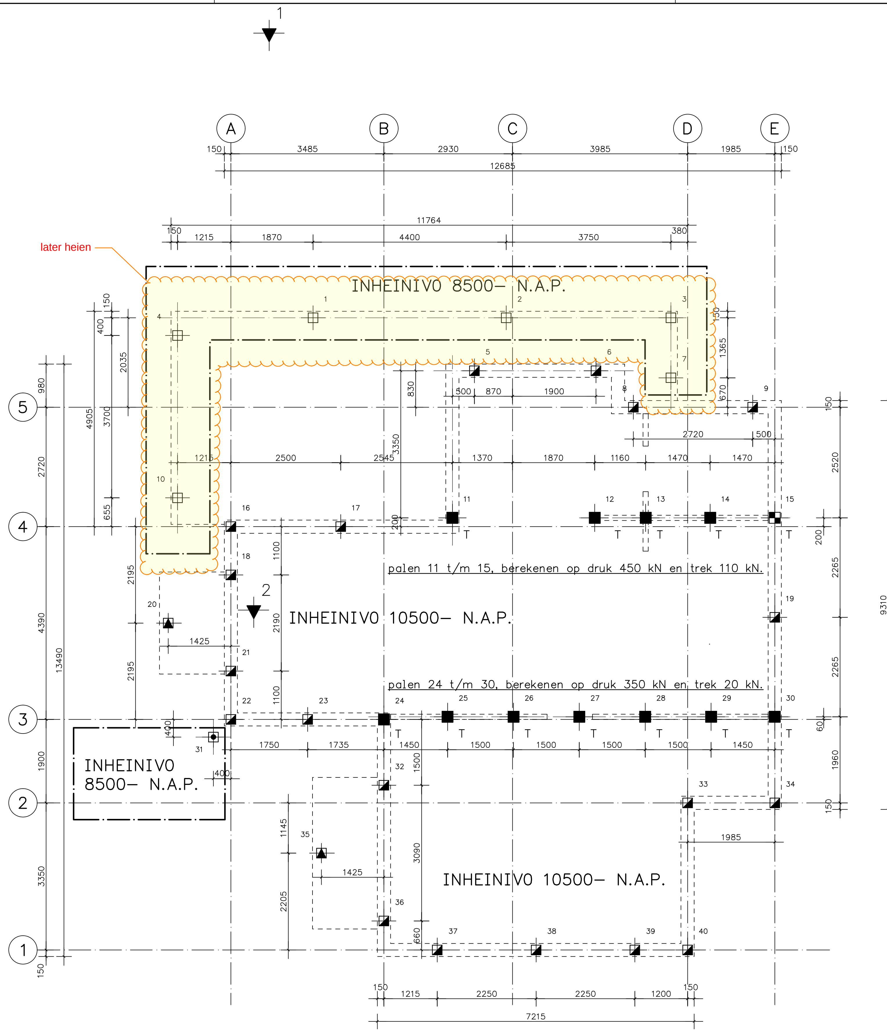
PALENPLAN.
