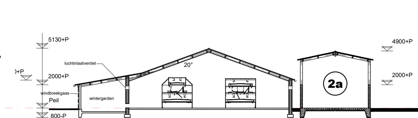
DOORSNEDE B-B GEBOUWNR 2 & 2a
