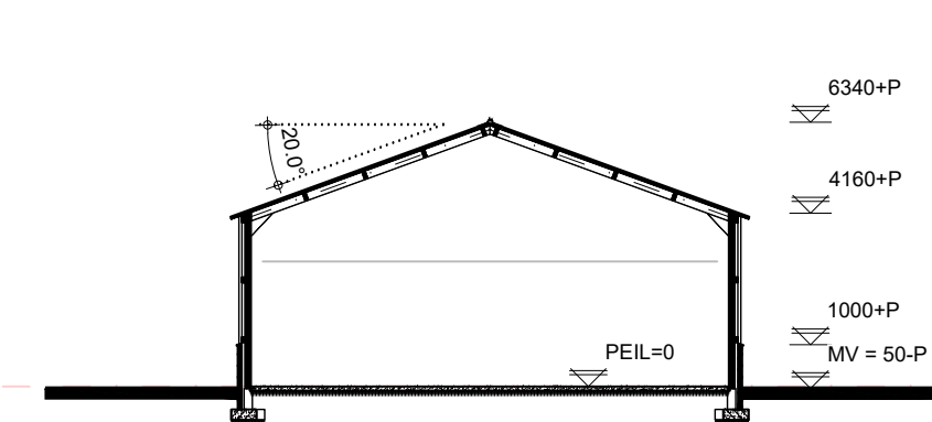
DOORSNEDE D-D GEBOUWNR 4
