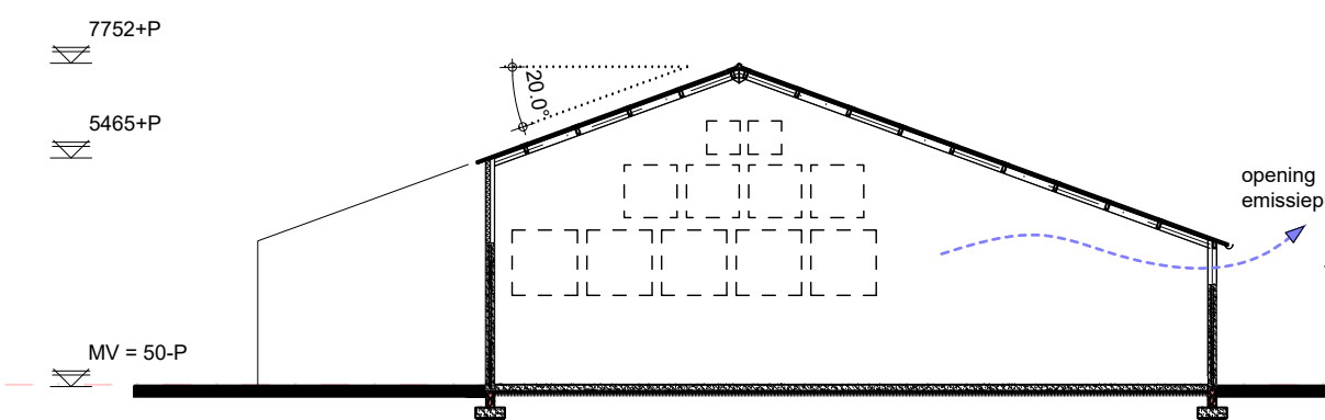
DOORSNEDE A"-A" GEBOUWNR 1
