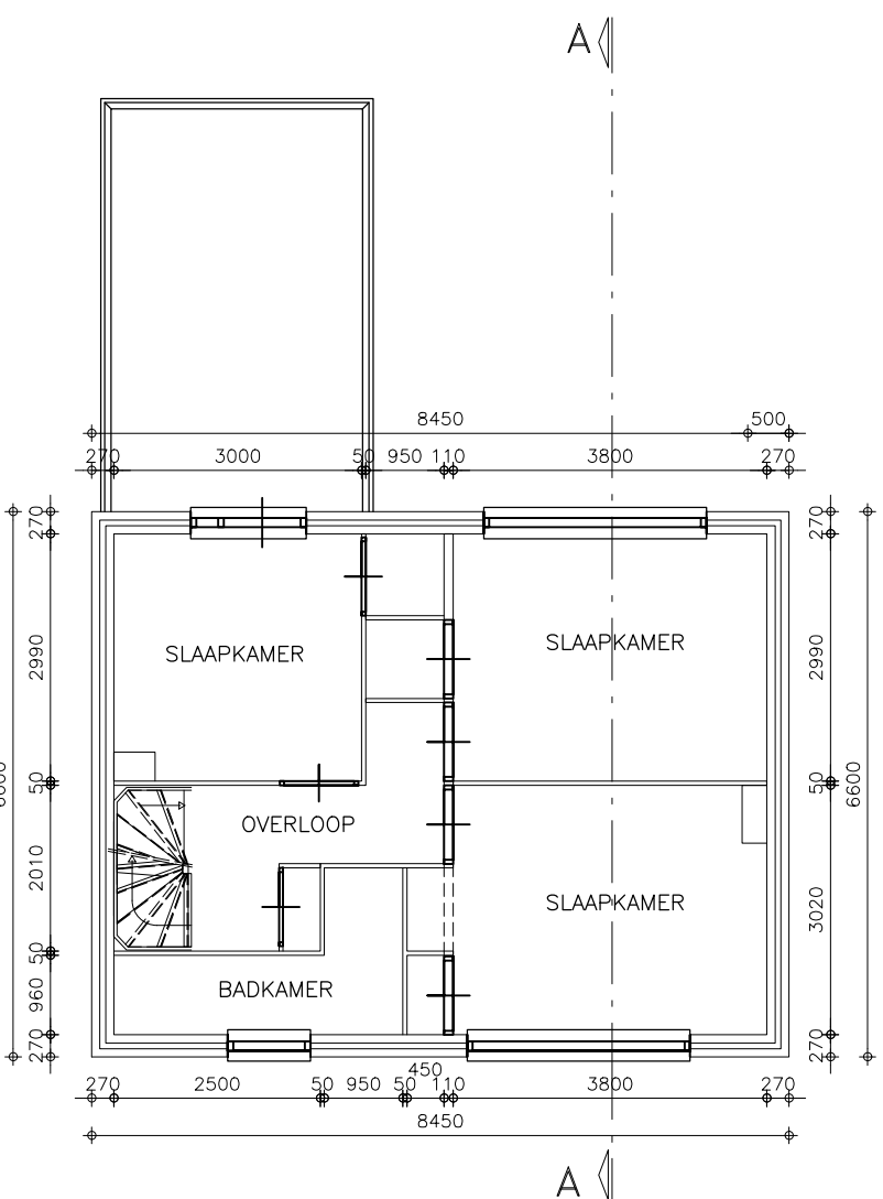
plattegrond 1e verdieping - bestaand
