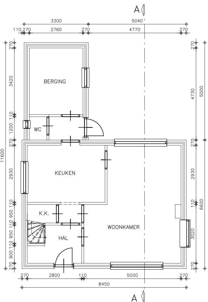
plattegrond begane grond - bestaand
