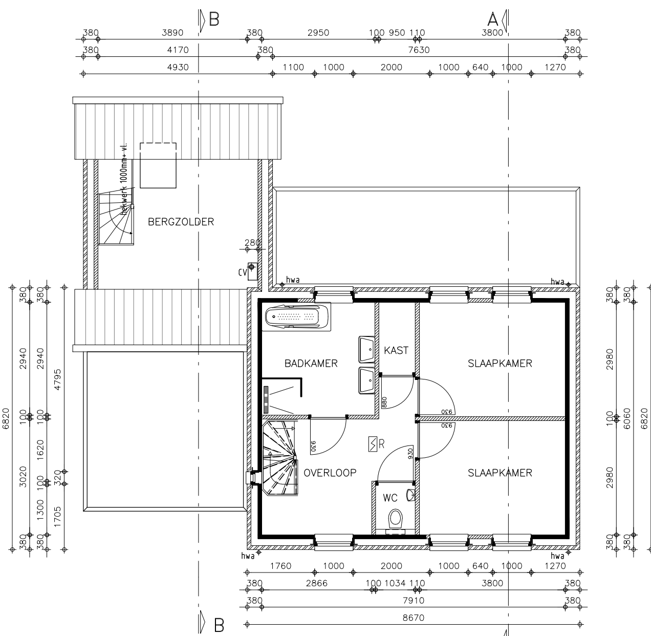
plattegrond 1e verdieping - nieuw
