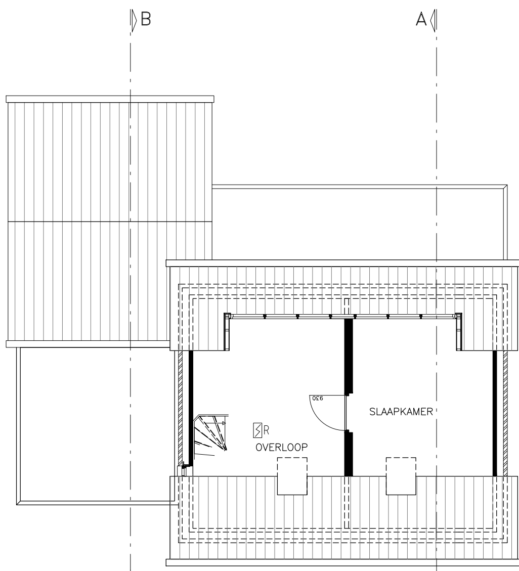
plattegrond zolder - nieuw
