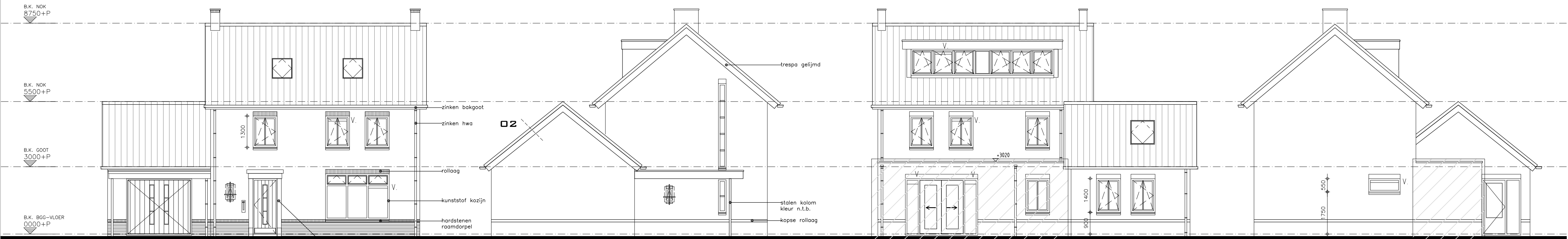
voorgevel - nieuw
