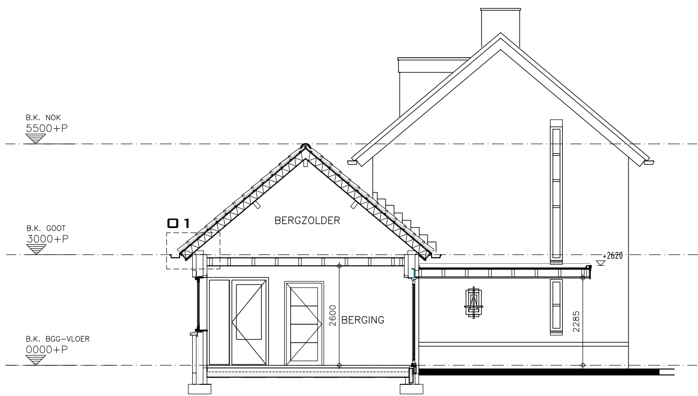
doorsnede BB
