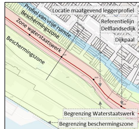
Figuur 13: Voorbeeld weergave: ligging van de Delflandsedijk op de leggerkaart
