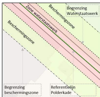
Figuur 18: Voorbeeld weergave: Ligging polderkade (zonder waterkerend kunstwerk) op leggerkaart en bijbehorend locatie specifiek leggerprofiel
