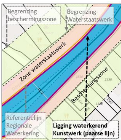
Figuur 19: Voorbeeld weergave: Ligging regionale waterkering (met waterkerend kunstwerk) op leggerkaart en bijbehorend locatie specifiek leggerprofiel
