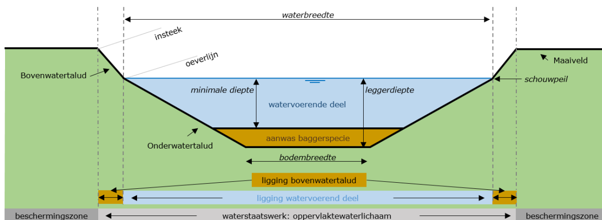
Figuur 23: Schematische weergave standaard trapezium leggerprofiel van een oppervlaktewaterlichaam.
