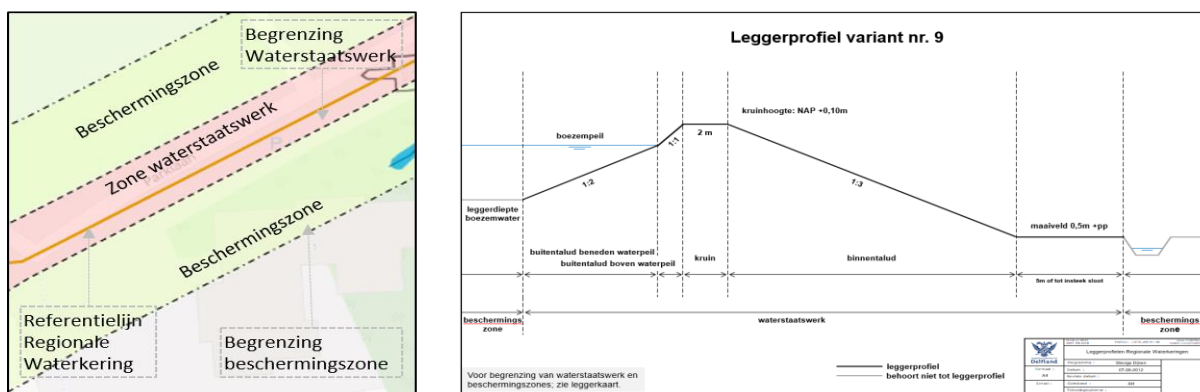
Figuur 16: Voorbeeld weergave: Ligging regionale waterkering (zonder waterkerend kunstwerk) op leggerkaart en bijbehorend locatie specifiek leggerprofiel
