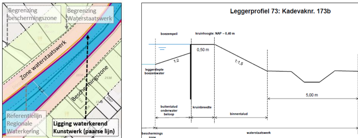
Figuur 17: Voorbeeld weergave: Ligging regionale waterkering (met waterkerend kunstwerk) op leggerkaart en bijbehorend locatie specifiek leggerprofiel
