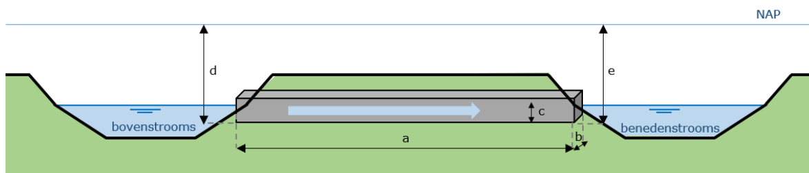
Figuur 37: Schematische weergave leggerprofiel van een duiker.
