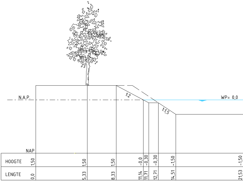
DOORSNEDE B-B
