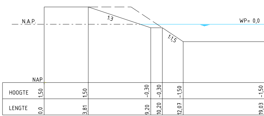
DOORSNEDE A-A
