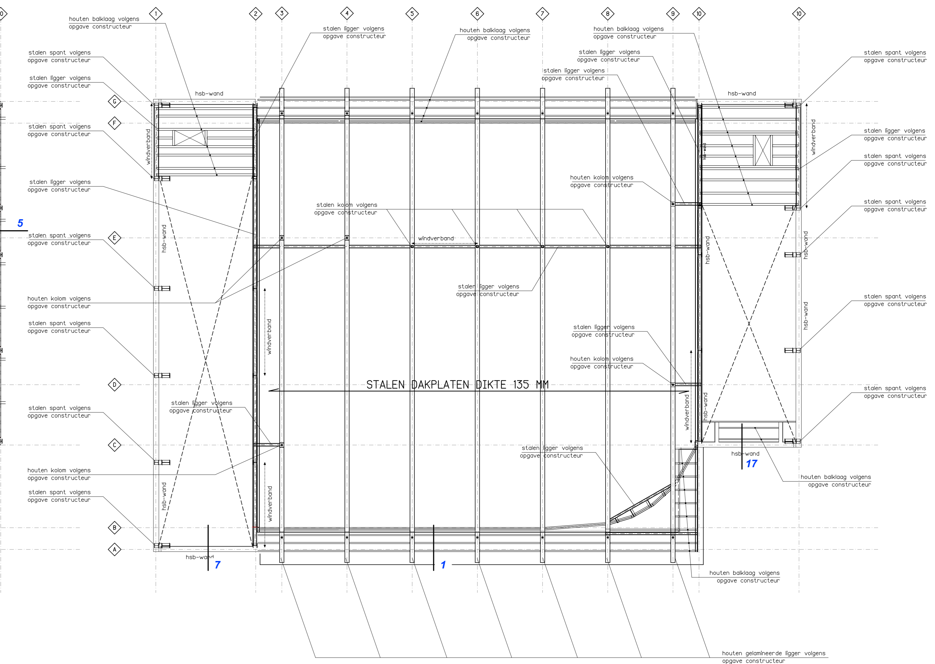
- 1E VERDIEPINGSVLOER -
