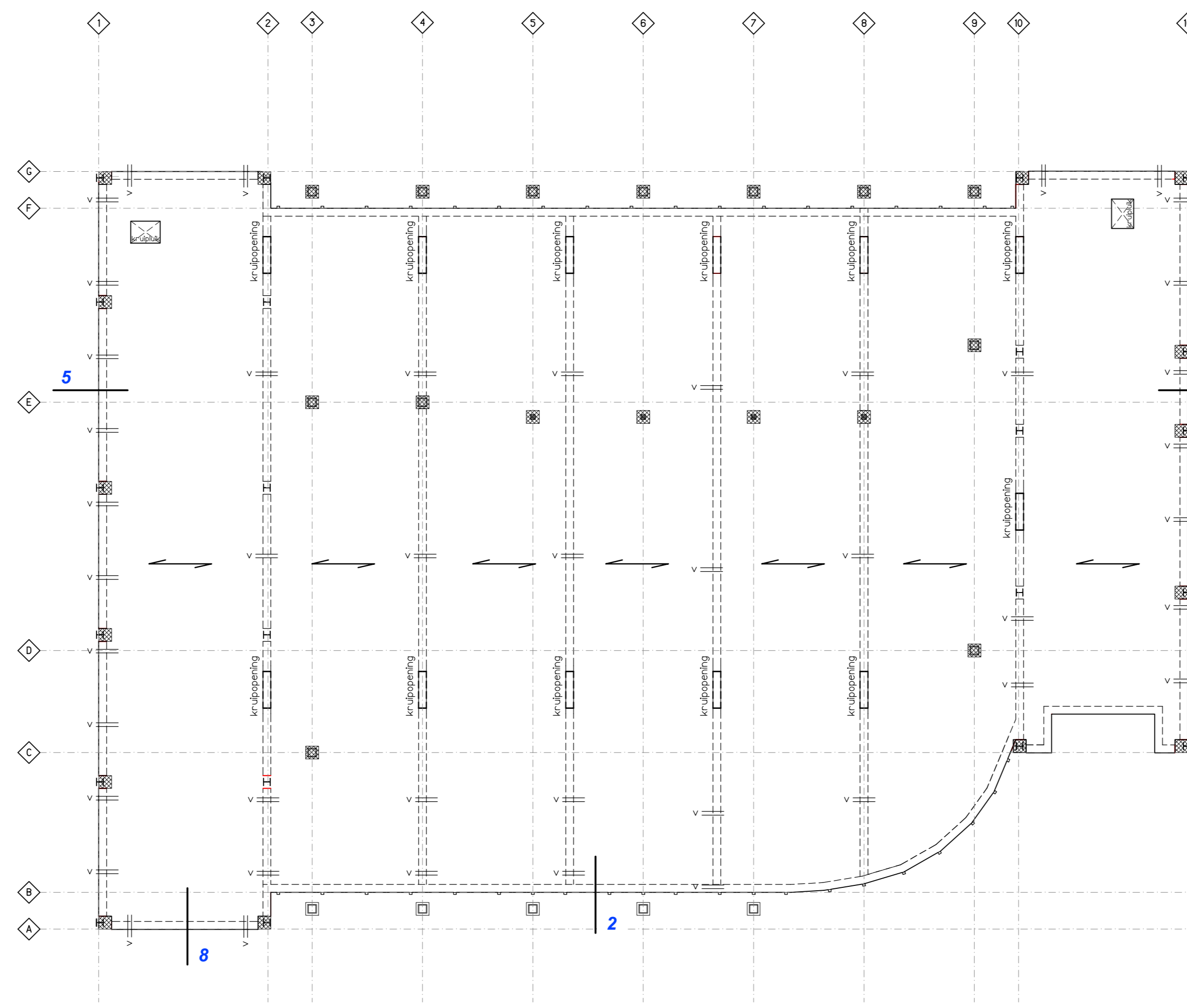
- BEGANE GRONDVLOER -
