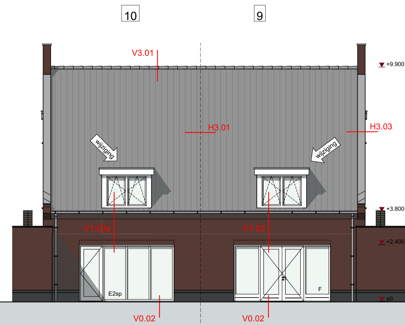
ACHTERGEVEL
