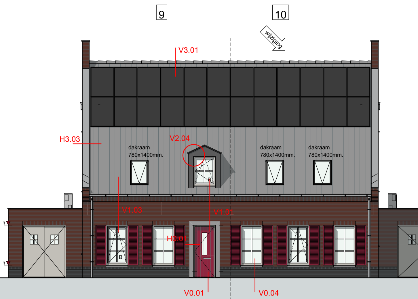
VOORGEVEL
