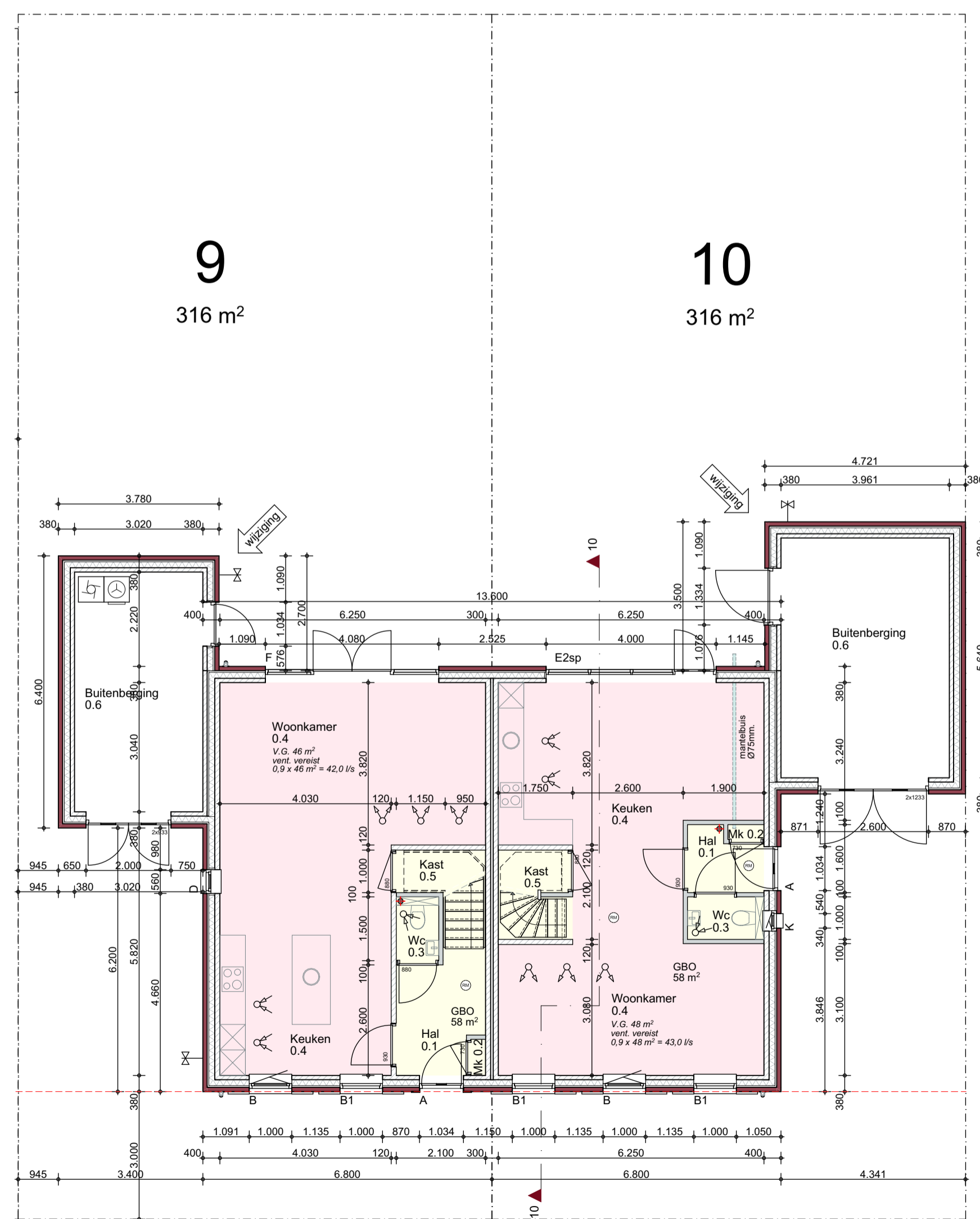
BEGANE GROND
