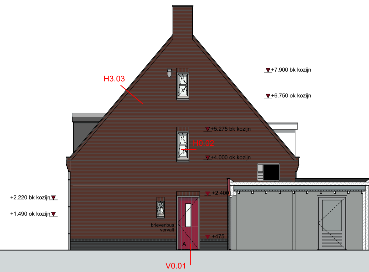
RECHTER ZIJGEVEL
