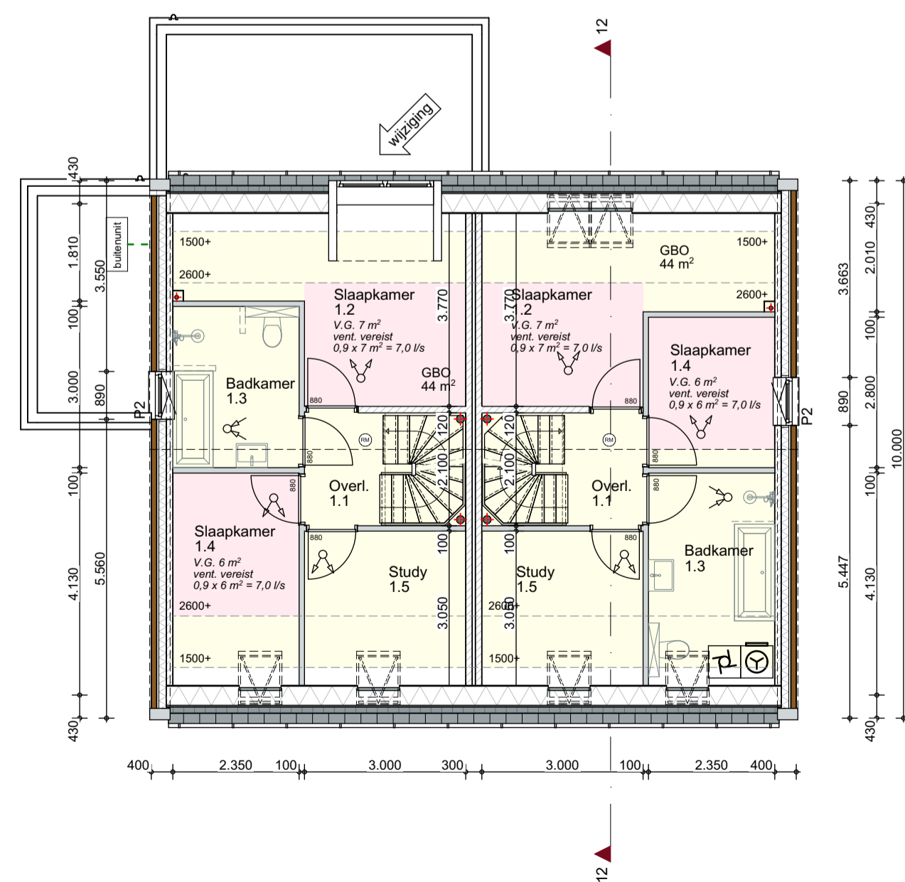
VERDIEPING
