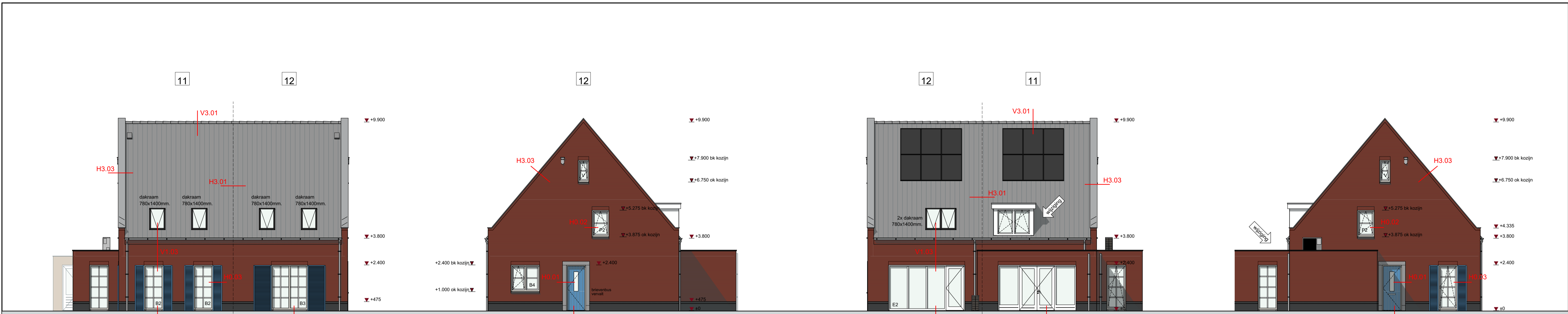
VOORGEVEL
