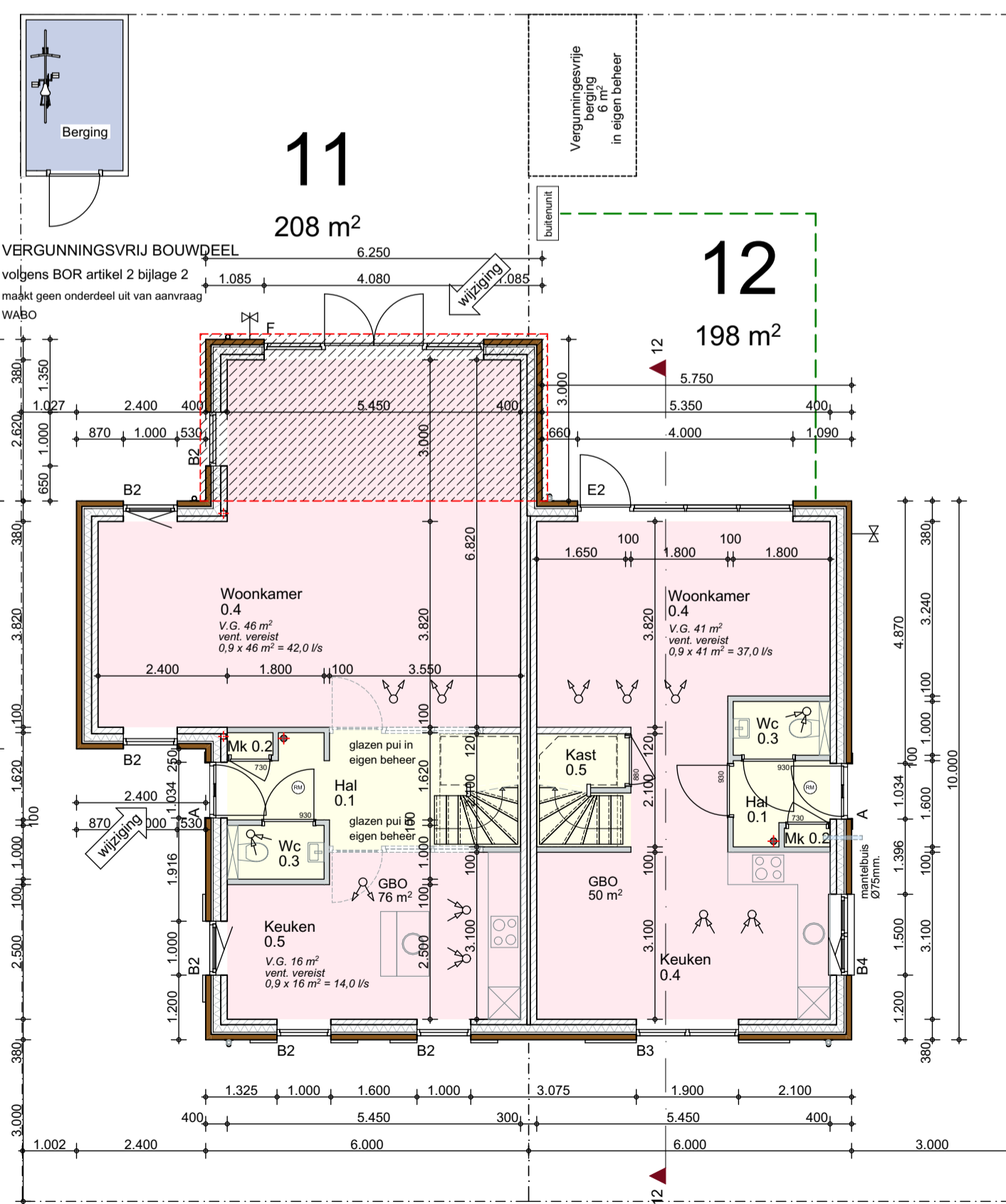
BEGANE GROND
