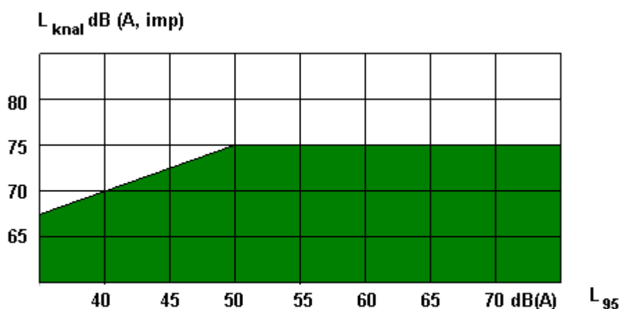
Grafiek uit Circulaire schietlawaai, mei 2006: Maxima van L_{\text{knal}} in relatie tot het omgevingsgeluid ( L_{95} ) ter voorkoming van schrikreacties
