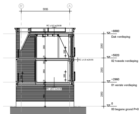
Doorsnede C-C
