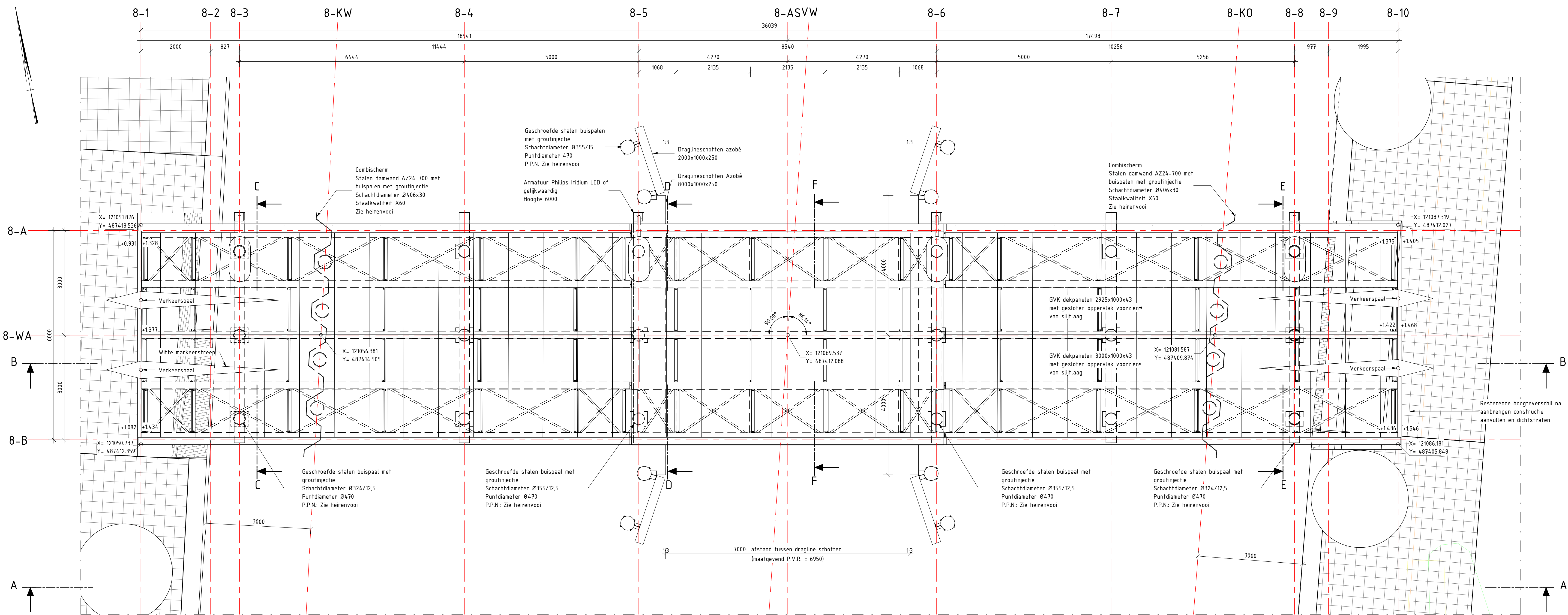
Bovenaanzicht Schaal: 1 : 50
