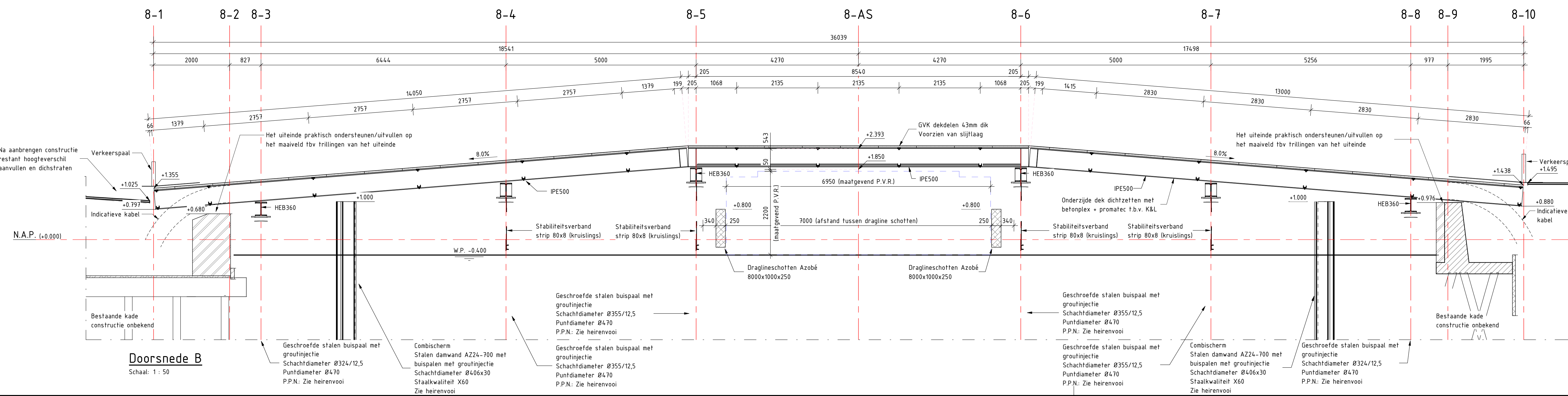
Aanzicht A Schaal: 1 : 50
