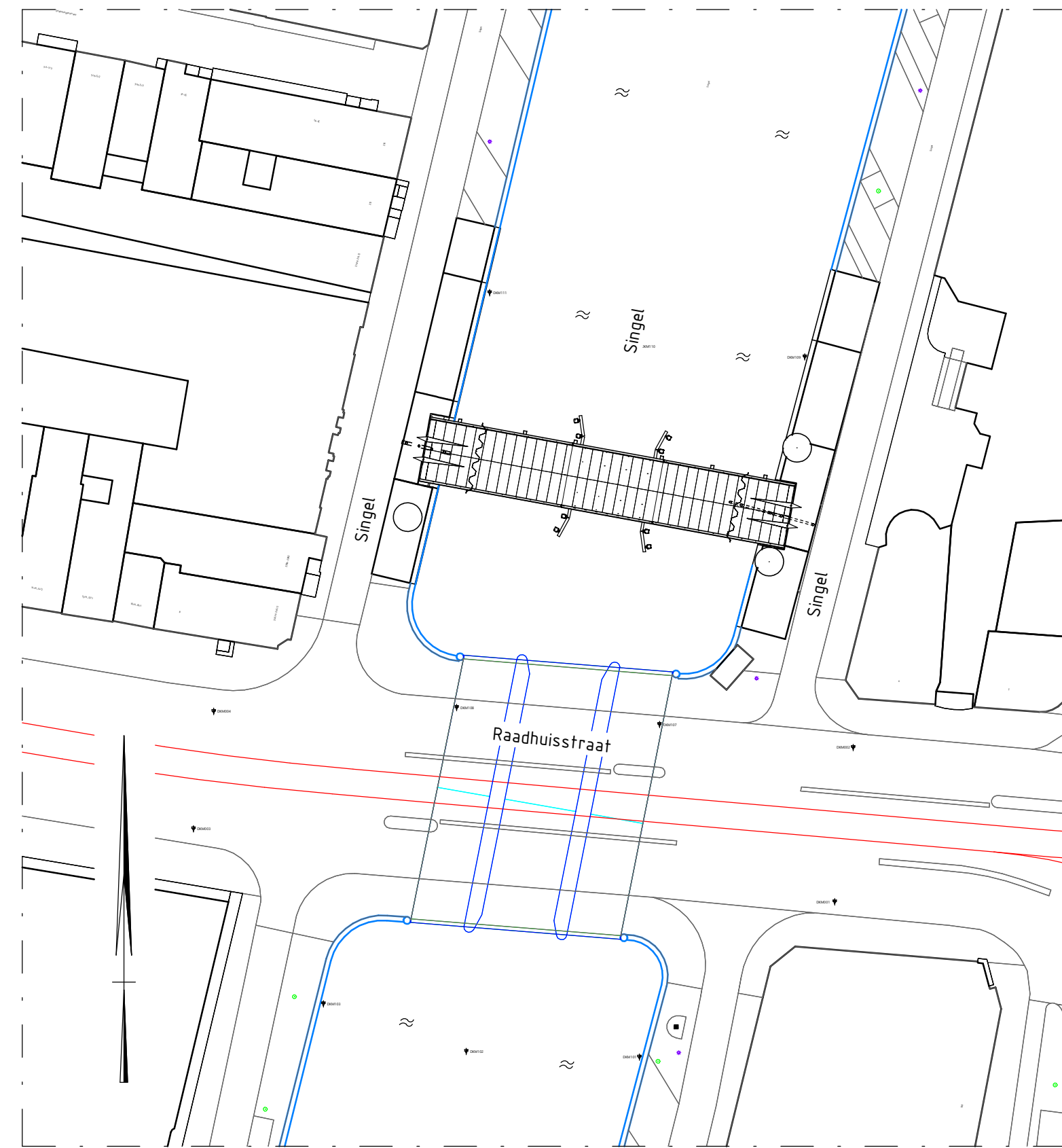
Situatie Schaal: 1 : 500
