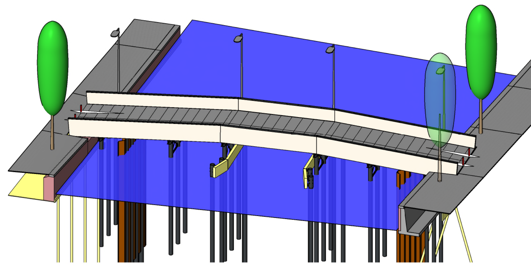
3D impressie Schaal:
