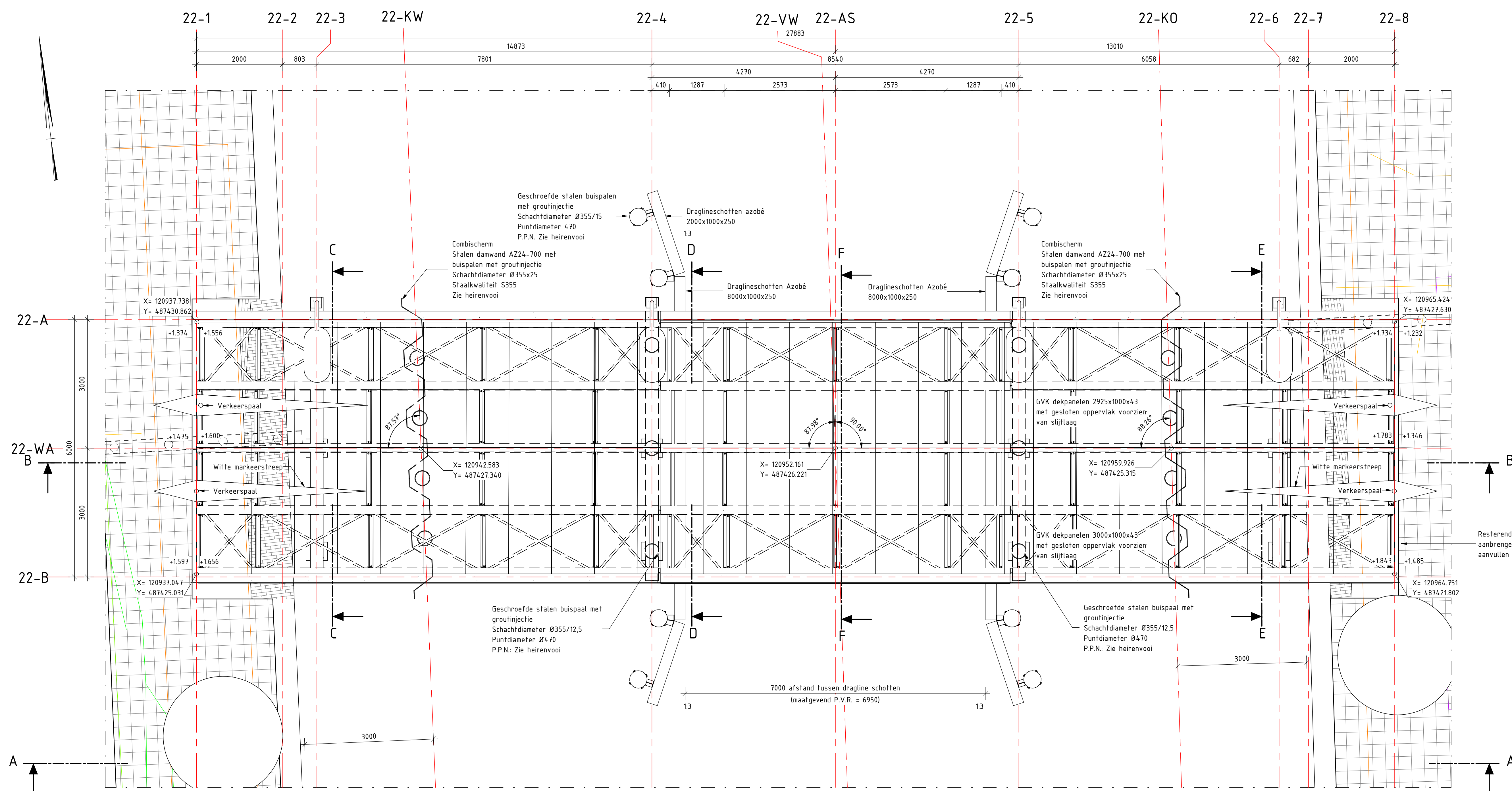
Bovenaanzicht Schaal: 1 : 50
