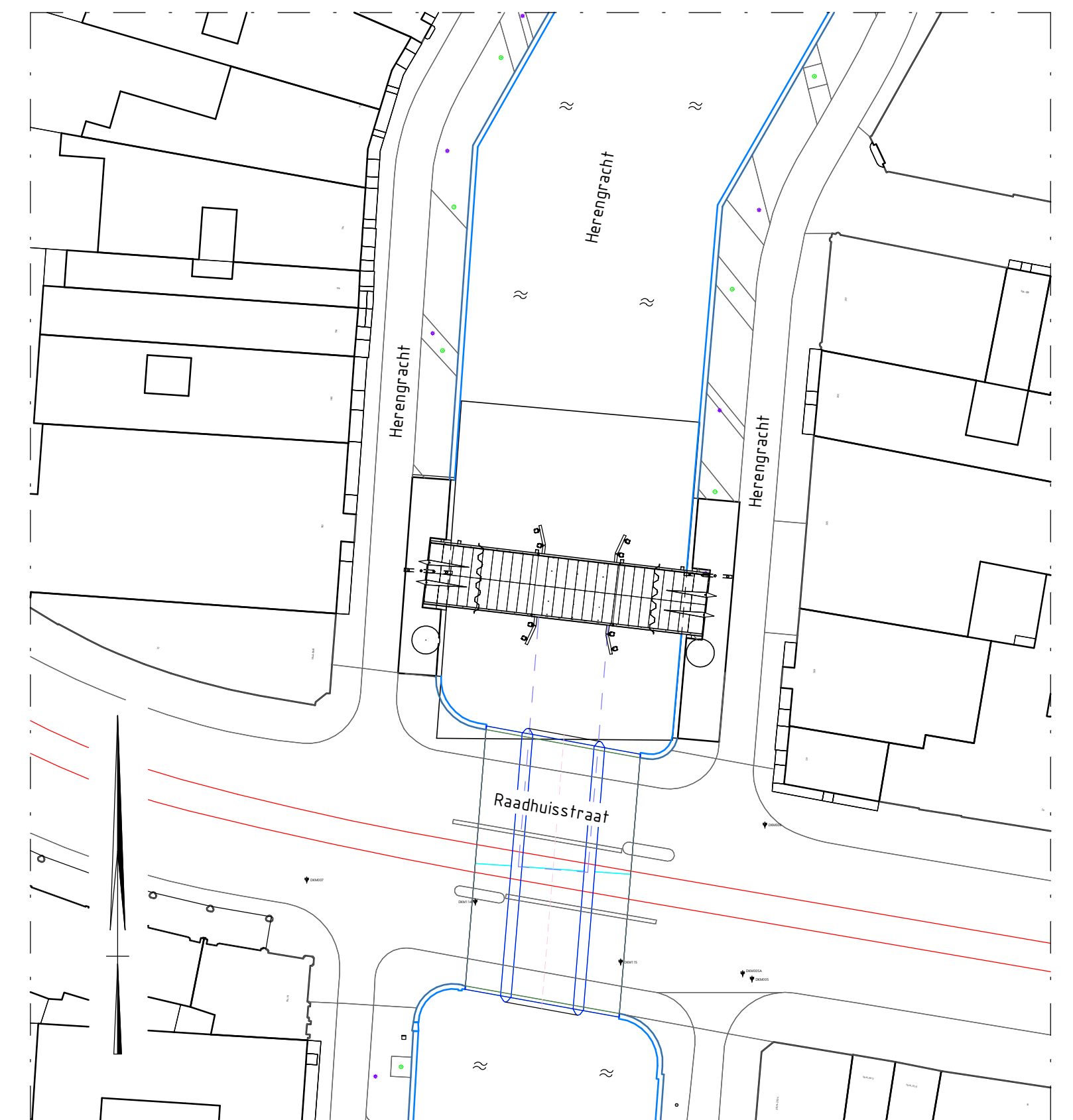
Situatie Schaal: 1 : 500
