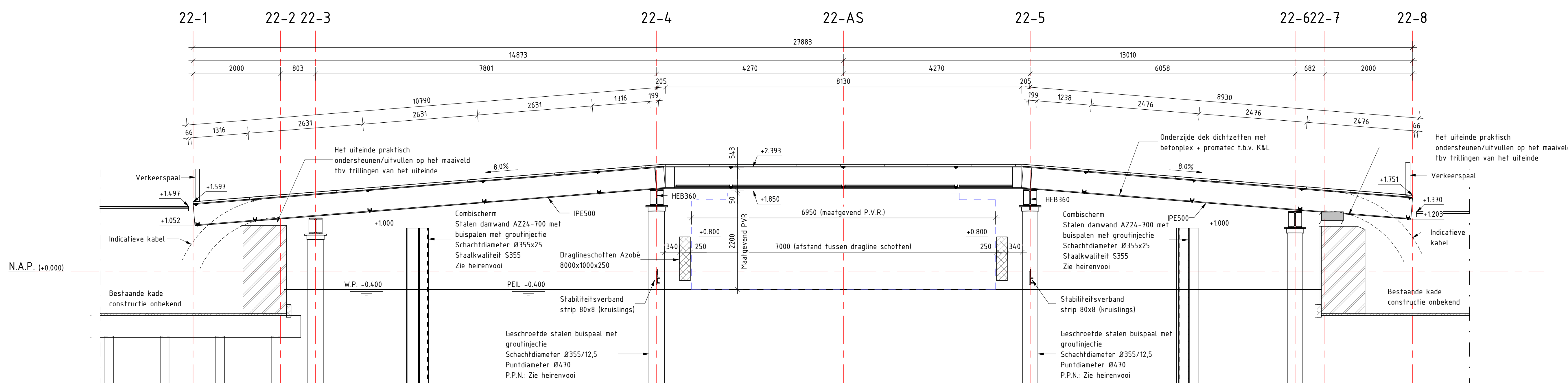
Doorsnede B Schaal: 1 : 50
