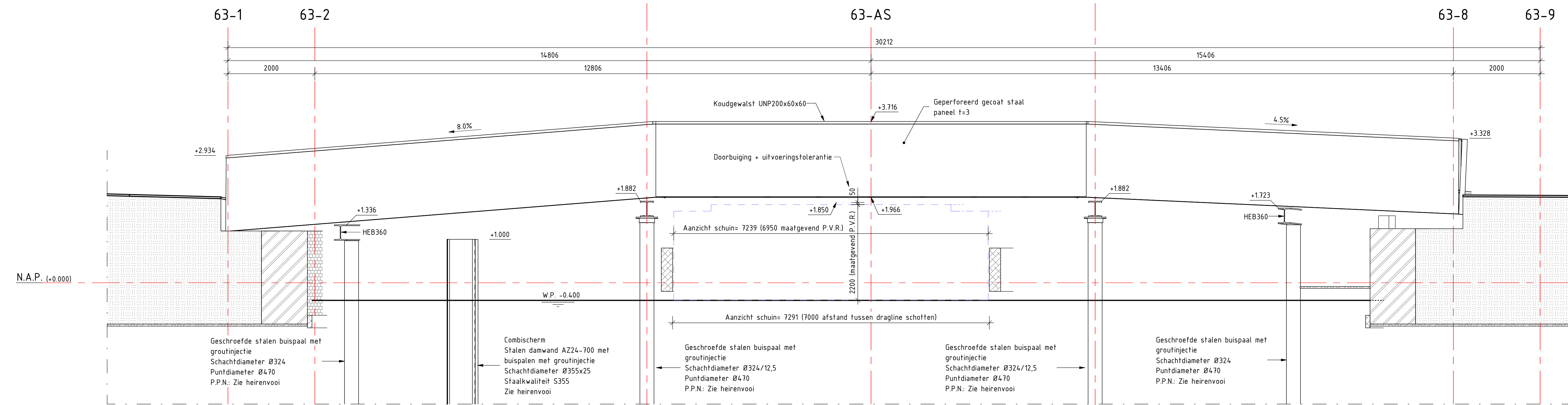
Aanzicht A Schaal: 1 : 50
