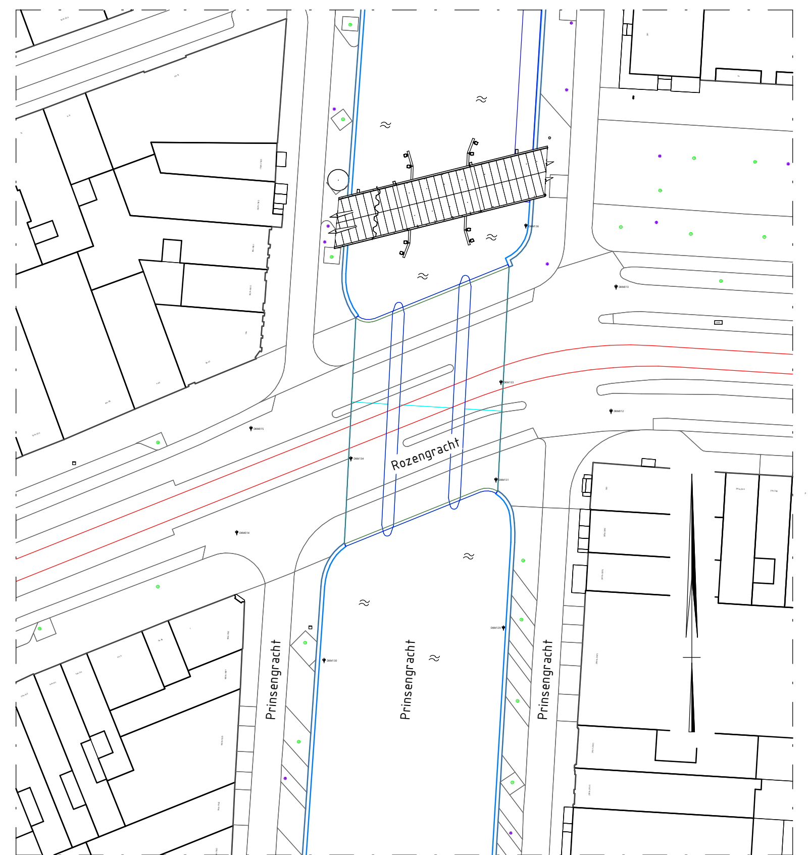
Situatie Schaal: 1 : 500
