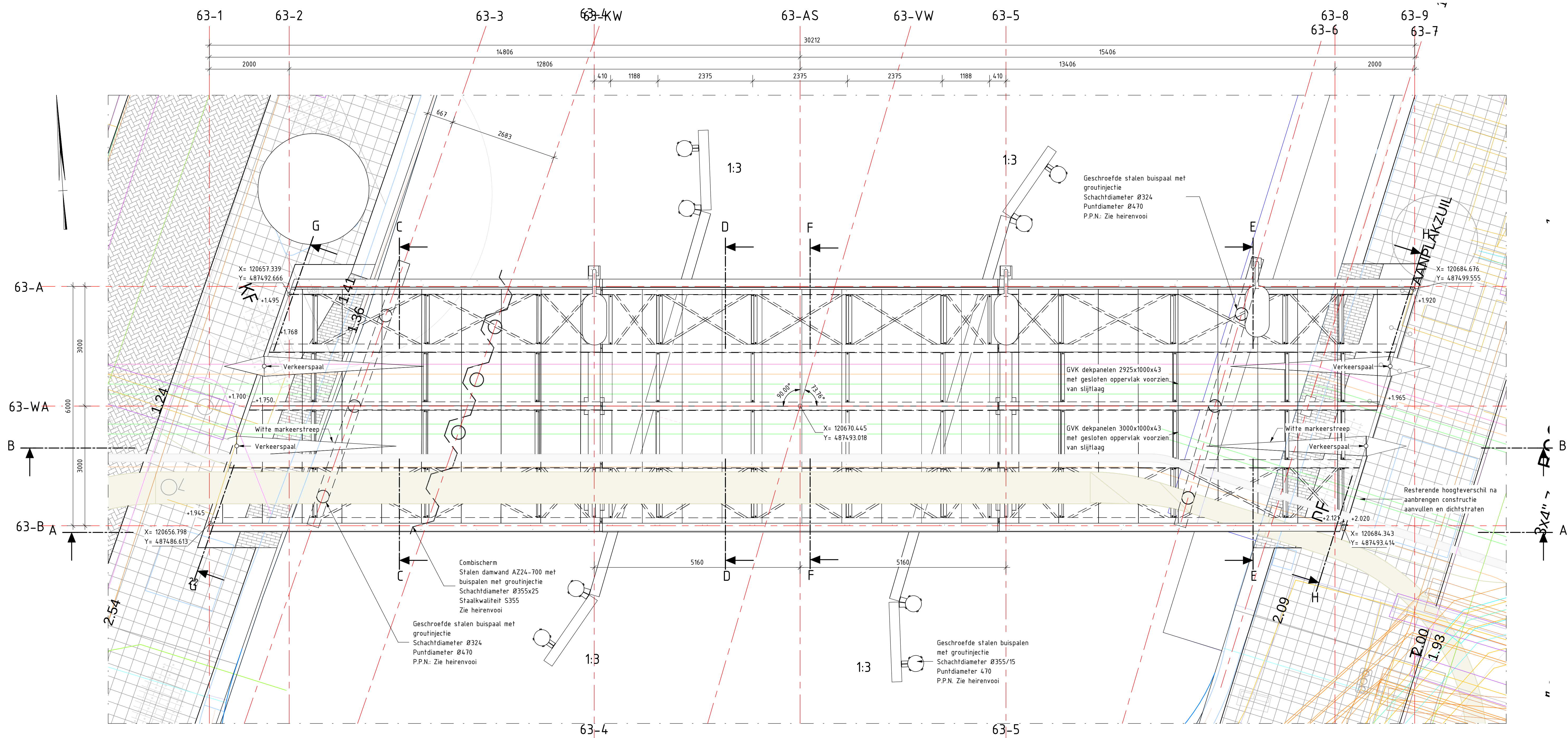
Bovenaanzicht Schaal: 1 : 50
