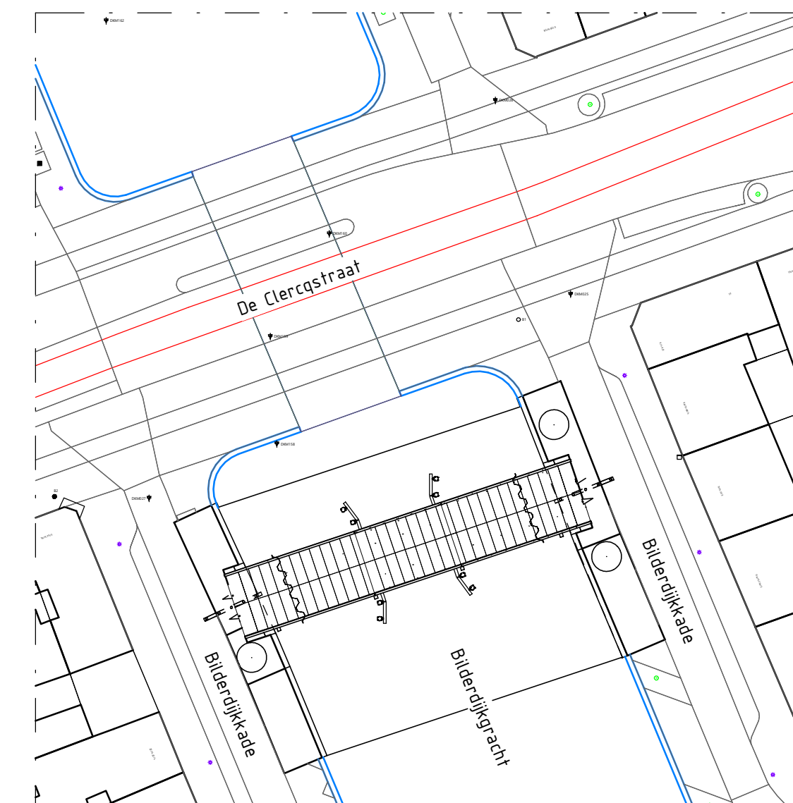
Situatie Schaal: 1 : 500
