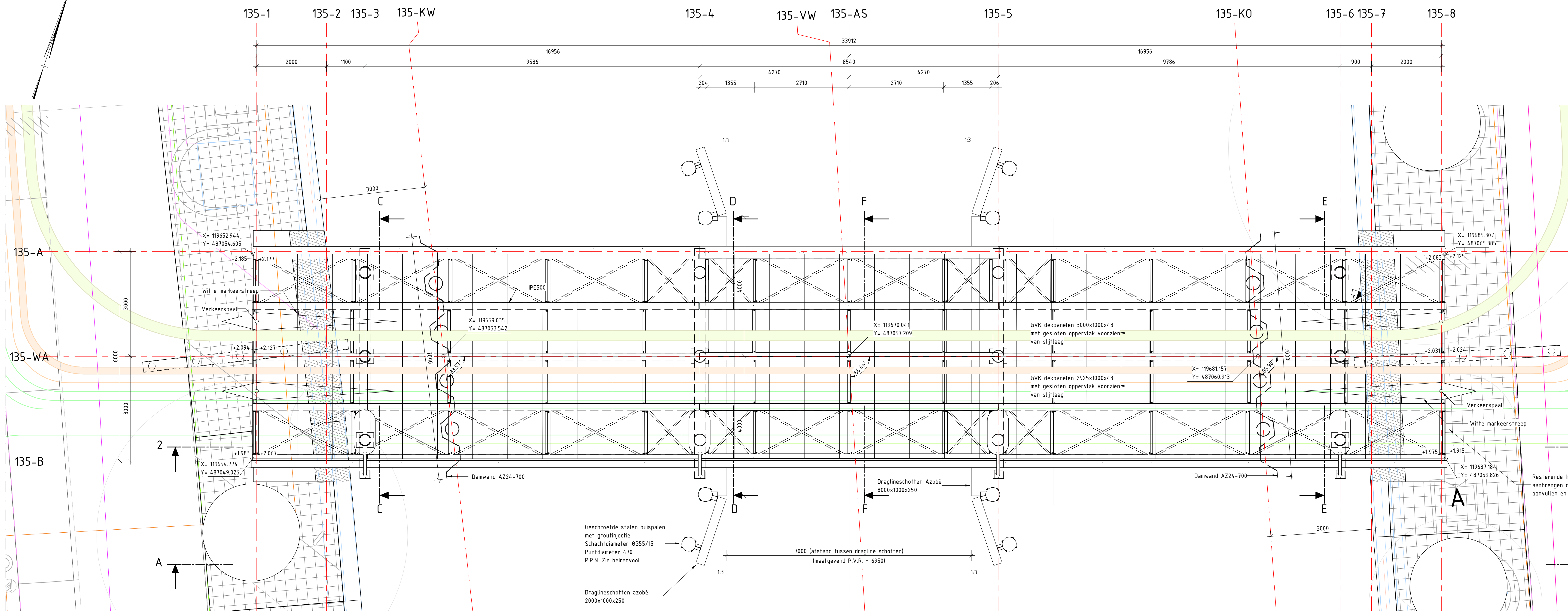
Bovenaanzicht Schaal: 1 : 50
