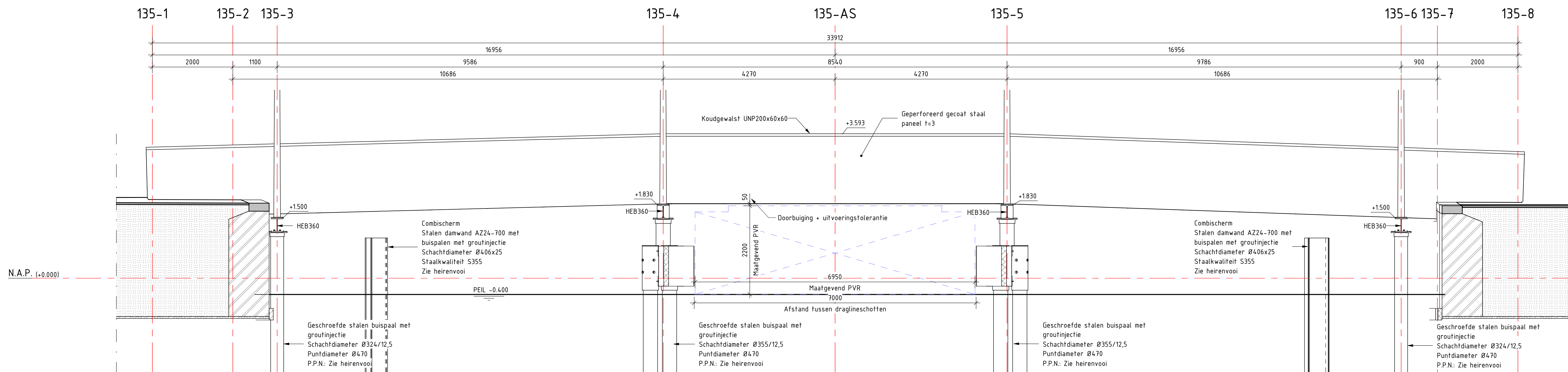
Aanzicht A Schaal: 1 : 50
