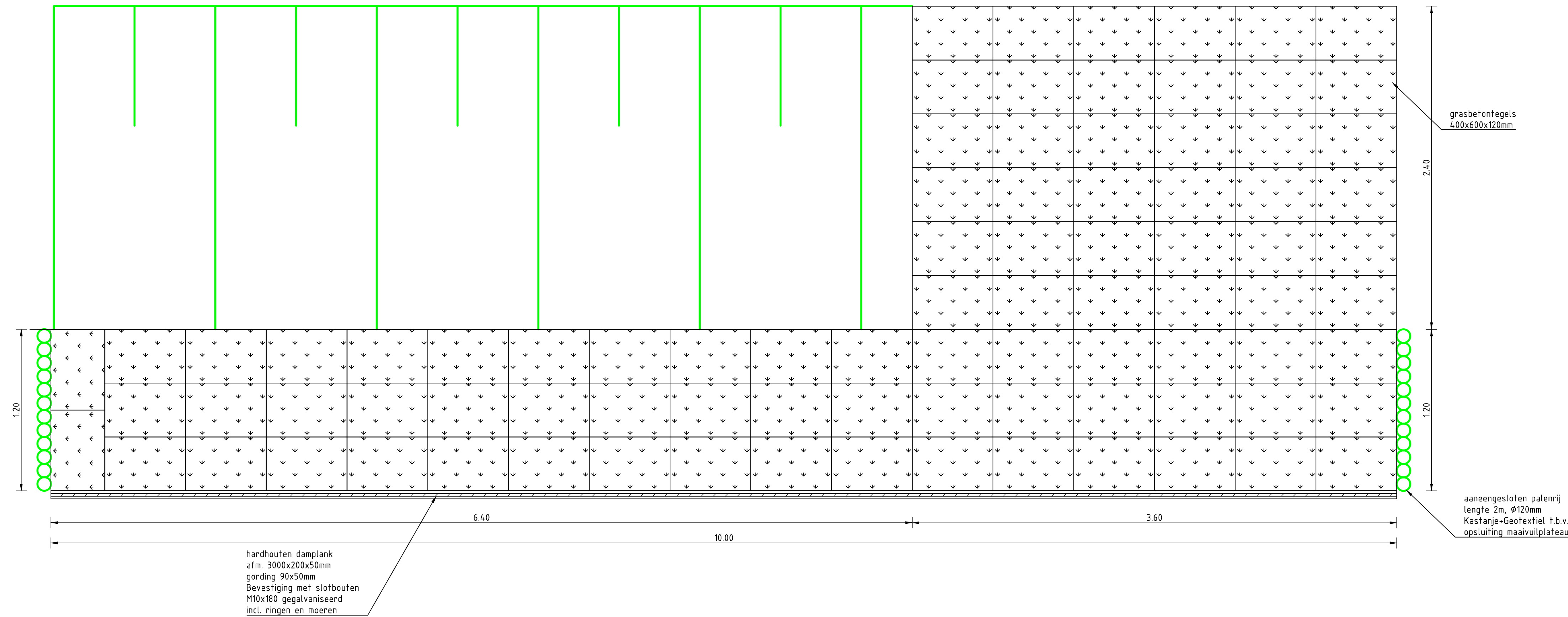
Bovenaanzicht maaiboot inlaatplaats schaal 1:20
