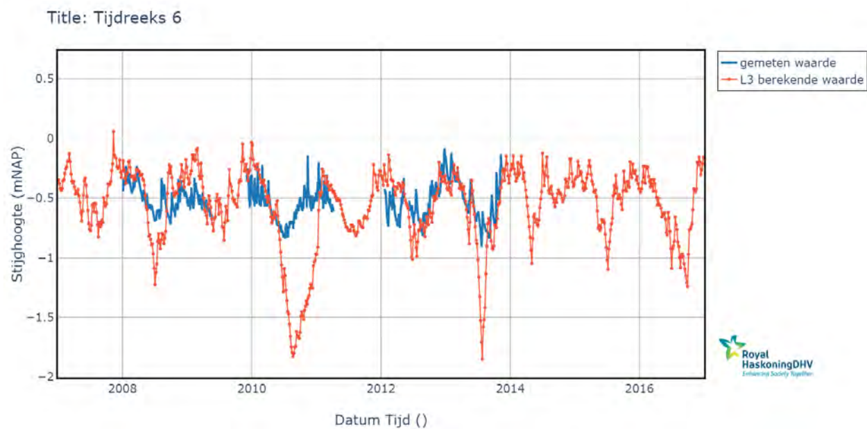
Figuur 5-3 Grafiek van model (rode lijn) en meting (blauwe lijn) voor peilbuis 6 (zie Figuur 4-4 voor de locatie van deze peilbuis).
