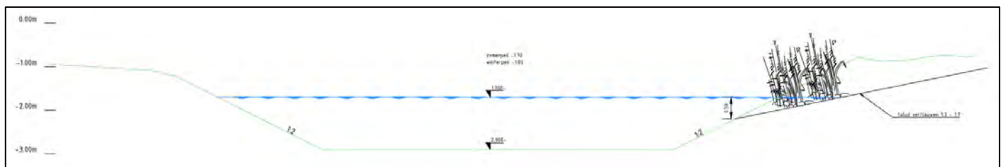
Figuur 11: dwarsprofiel van de aan te leggen natuurvriendelijke oever. Het talud wordt verflauwd naar een helling van 1:3 -1:7.
