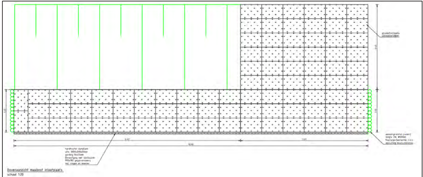
Figuur 9: Bovenaanzicht maaiboot inlaatplaats bij de Langeweg.
