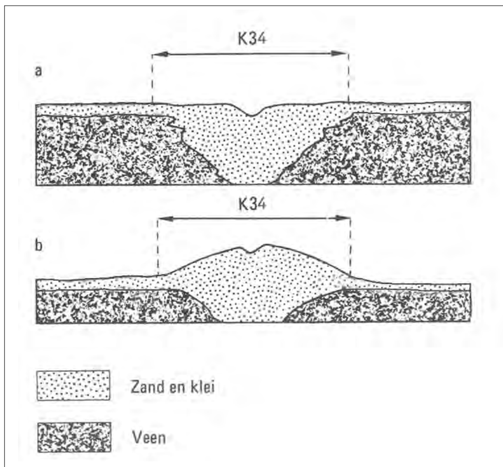
Figuur 3. Inversie van de hoogteligging rond een getij-oeverwal (K34; naar Stiboka & RGD, 1977).
