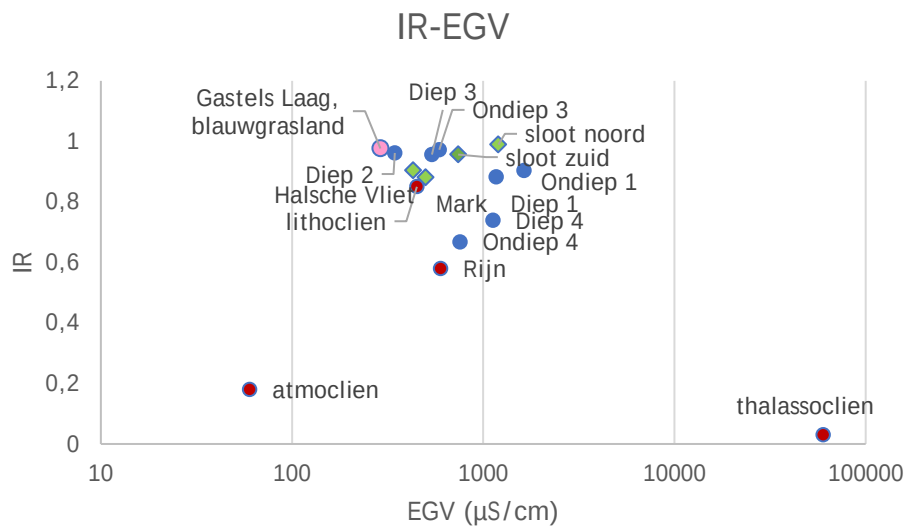
Figuur 10. IR-EGV-diagram van de grondwatermonsters (blauw), de oppervlaktewatermonsters (groen) en ter referentie atmoclien, thalassoclien en gemiddeld lithoclien water en gemengd oppervlaktewater (Rijn) (rood) en het grondwater dat in het blauwgrasland in het Gastels laag omhoog komt (roze). 'Ondiep' en 'diep' geven aan of het water uit het ondiepere of het diepere filter afkomstig was. Beide betreft ondiep grondwater.
