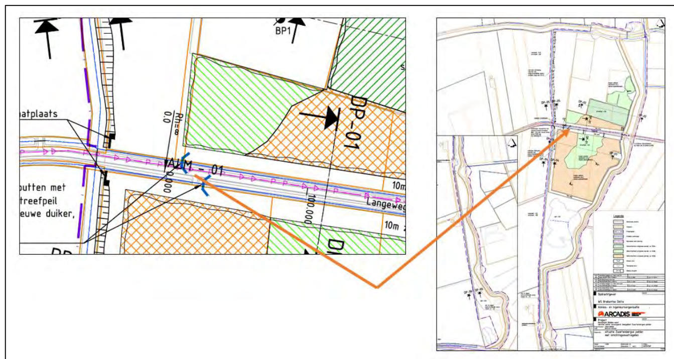
Figuur 8: Locatie twee nieuwe stuwputten in de A-watgangen aan weerskanten van de Langeweg: in detail (links) en op de overzichtstekening van het plangebied (rechts – zie oranje pijl )
