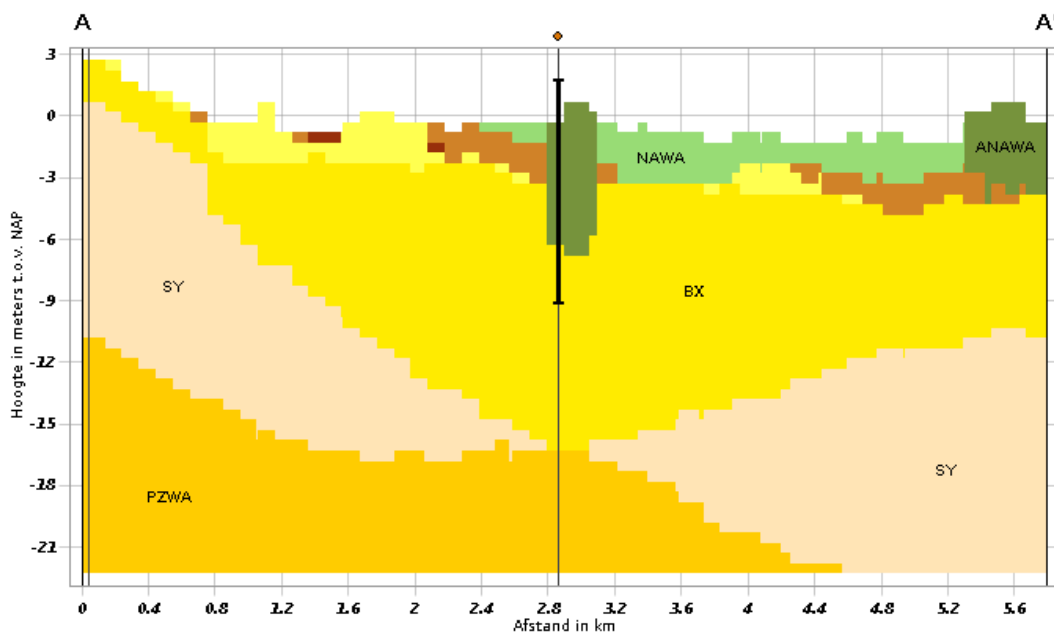
Figuur 2.3. Geo(hydro)logische doorsnede o.b.v. GEOTOP v1.4 ( www.dinoloket.nl ; mrt-2021) van Etten-Leur west via Kelsdok-Zwermlaken en de Zwartenbergese polder naar de Mark. PZWA = Peize & Waalre, SY= Stramproy, BX= Boxtel, NAWA = Naaldwijk-Walcheren, ANAW, Donkerbruin = Formatie van Nieuwkoop, Basisveen, Lichtbruin= Formatie van Nieuwkoop, Hollandveen.
