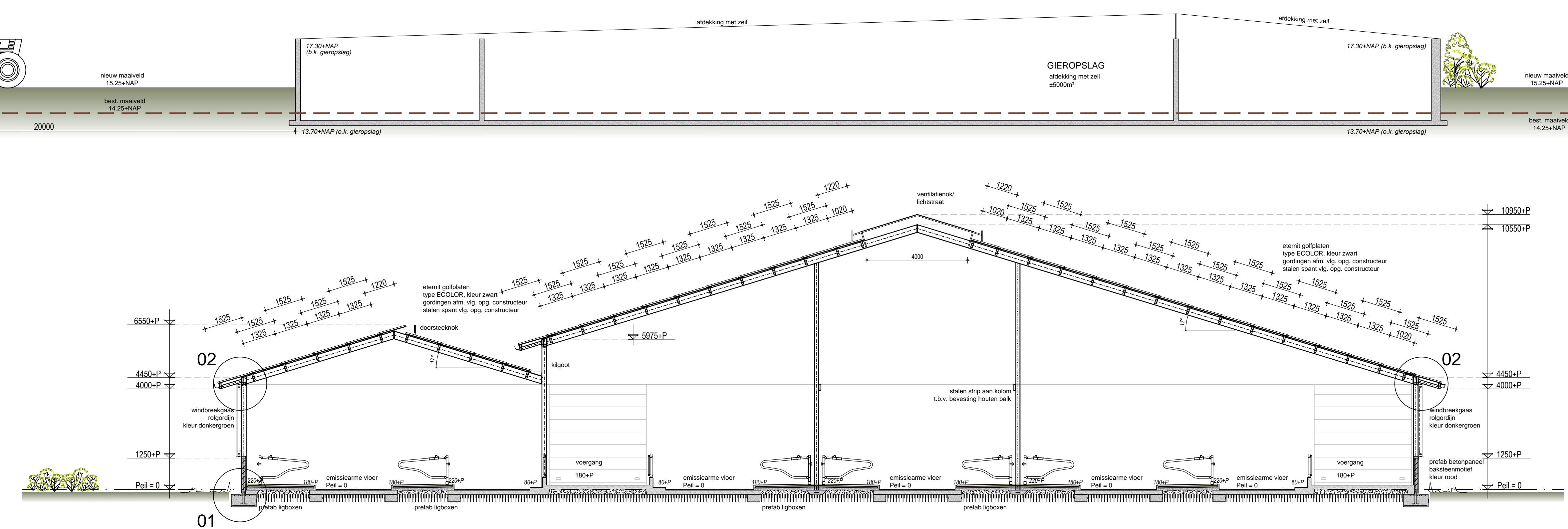
DOORSNEDE A-A
