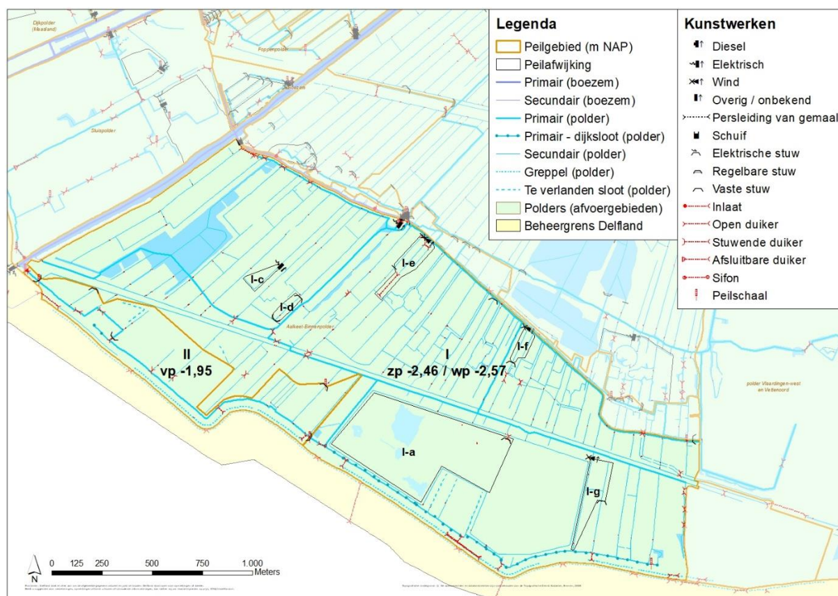
Figuur 4.4 Watersysteem
