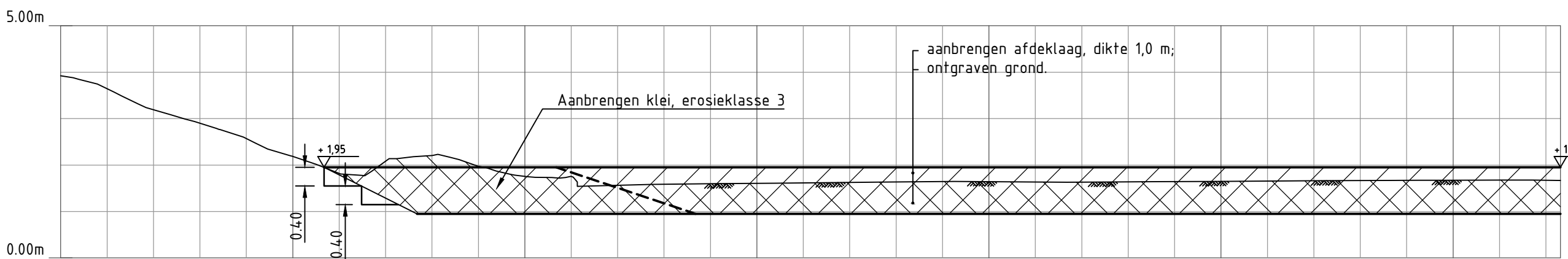
DWARSPROFIEL 3 Schaal 1:100
