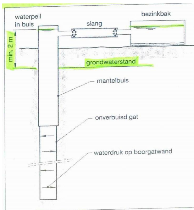
Figuur 12.4 Grondwaterpeil en waterpeil in boorgat.
