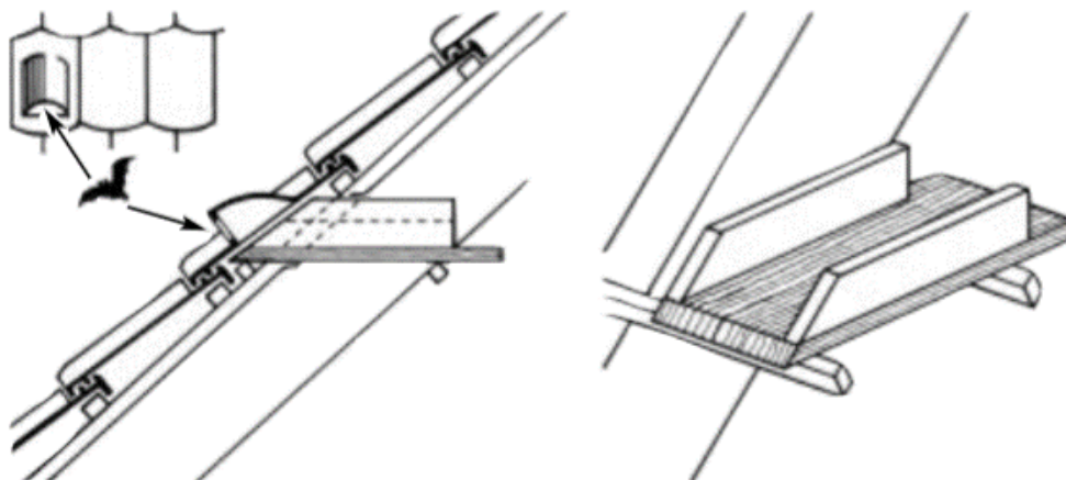
Figuur 14 Voorbeeld van een dakkast voor vleermuizen. Waarbij een opening in het dak toegang biedt tot een kast aan de binnenzijde van het dakbeschoot. Bron: Fledermaus Schutz im Siedlungsbereich, Deutscher Verband für Landschaftspflege.
