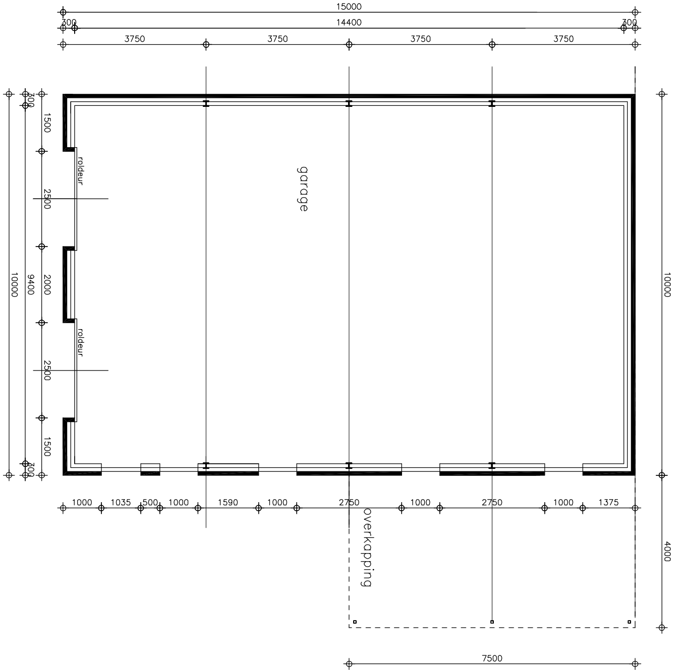
begane grond bestand
