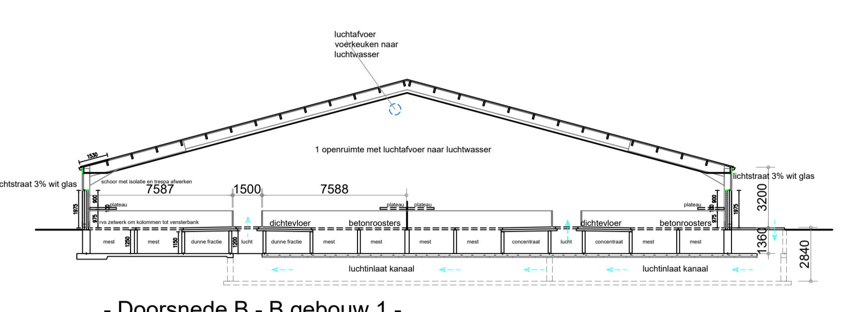
- Doorsnede B - B gebouw 1 -
