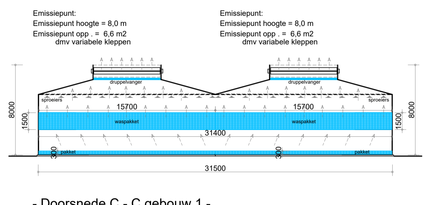
- Doorsnede C - C gebouw 1 -
