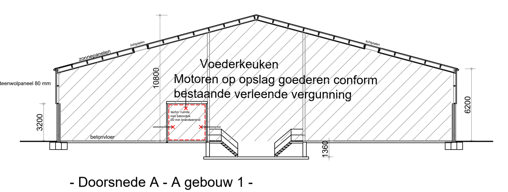
- Doorsnede A - A gebouw 1 -
