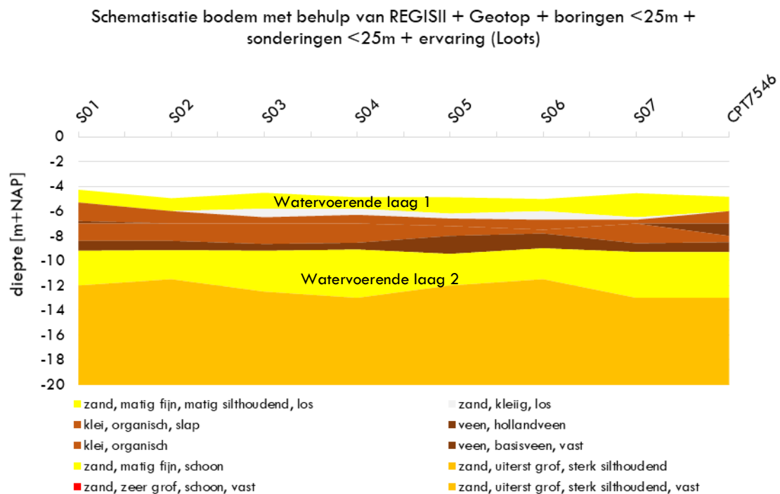
figuur 2 – schematisering bodem
