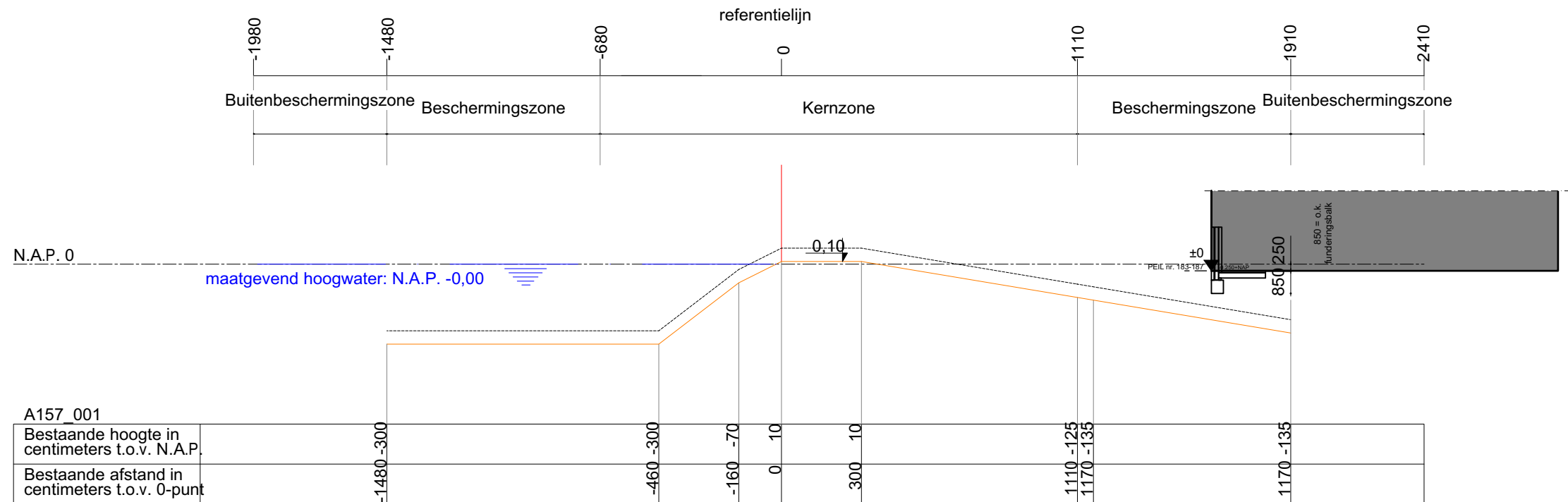
PROFIELDOORSNEDE kering: A157-001 schaal: 1a200
