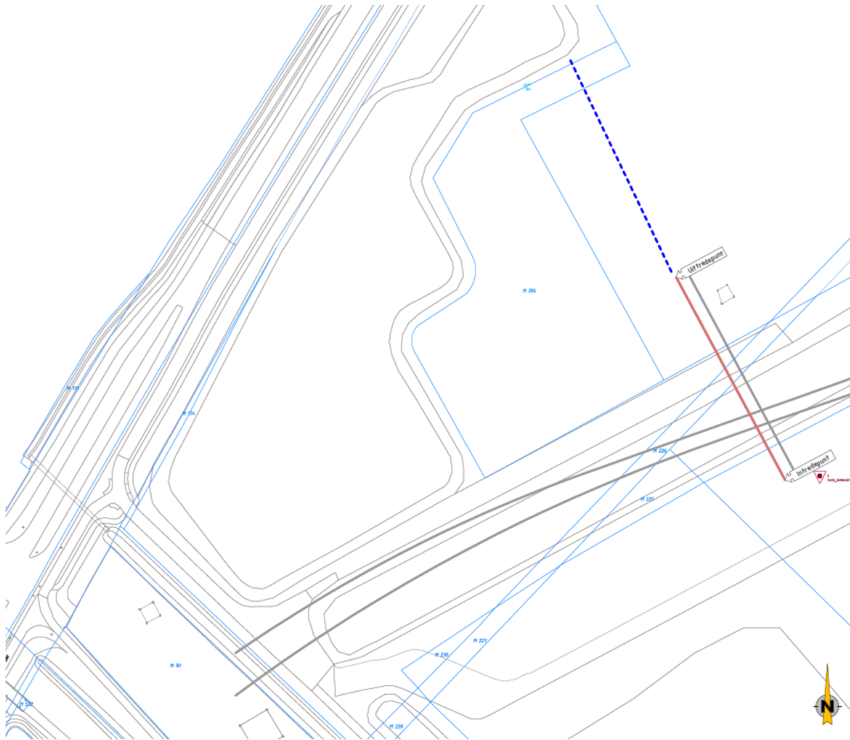
Figuur 1: De rode lijn geeft de locatie weer van de gestuurde boring.
