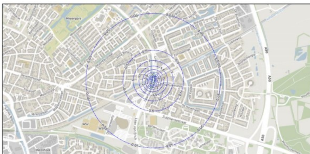
Figuur 13 – Maximale verlagingcontouren grondwaterstand [m] t.o.v. omgeving a.g.v. stationaire onttrekking.
