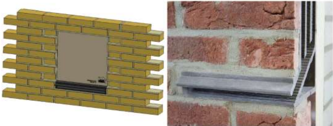
Figuur 4. Permanente vlemuiskast (3 x 4 stuks) als kraamverblijfplaats. Merk Tichelaar, type 'groot' of vergelijkbaar.
