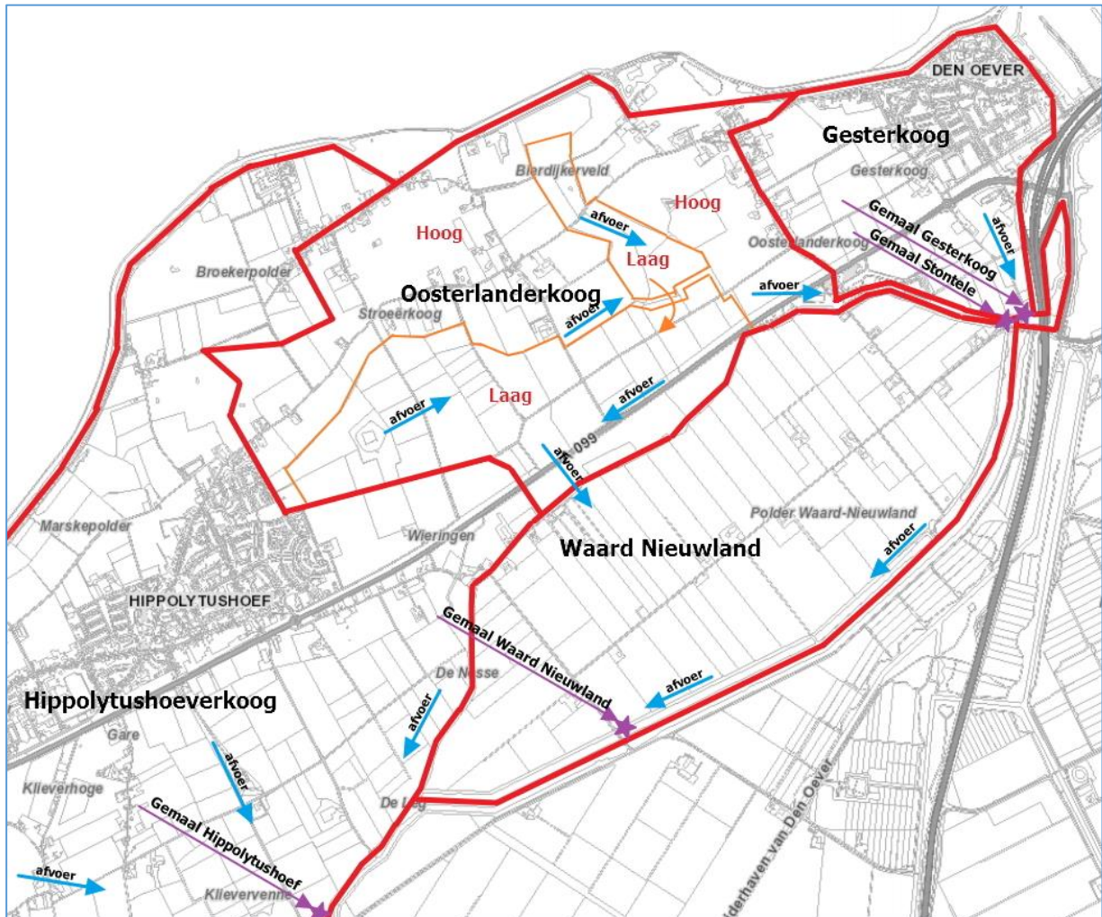
Figuur 1: Afvoerverdeling naar de diverse gemalen
